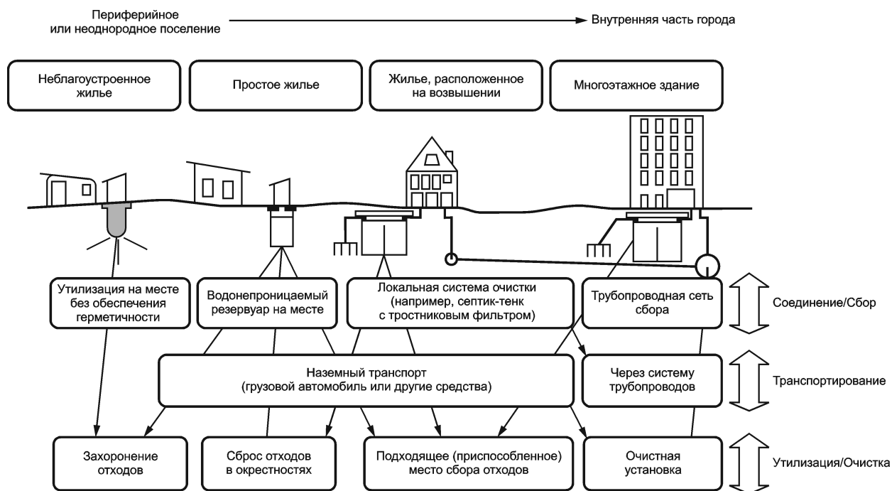
Рисунок В.2 — Типы систем удаления сточных вод
