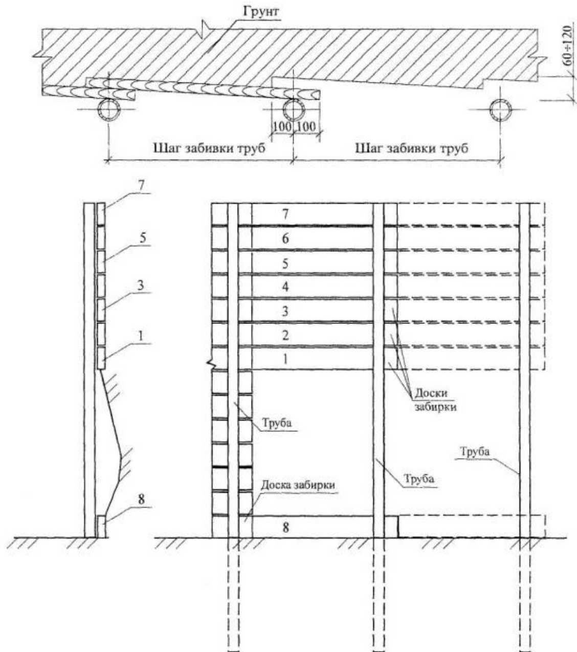
Рисунок 11 - Последовательность и схема устройства забирки
