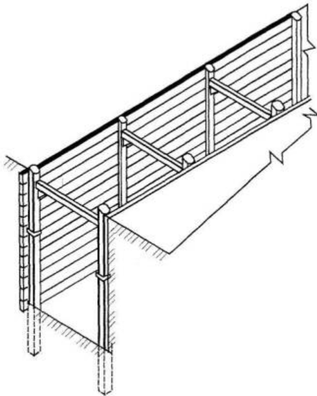
Рисунок 2 - Общая схема траншеи с верхним креплением
