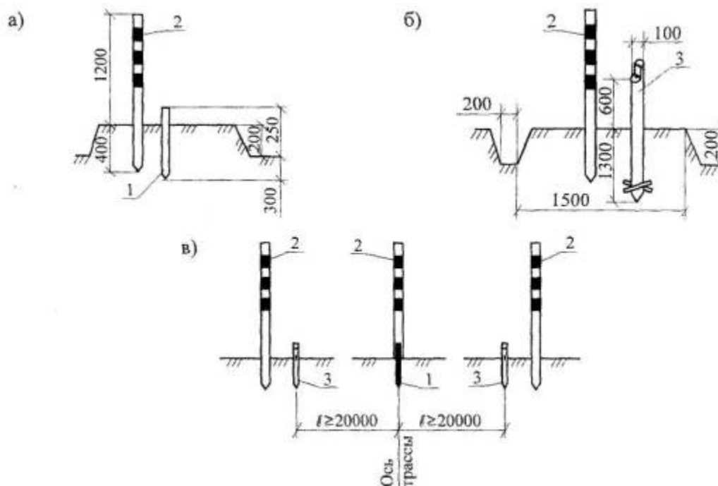
а, б - геодезические знаки; в - схема закрепления знаков разбивочных осей 1 - временный знак из дерева или металла \varnothing 15-30 мм; 2 - опознавательная веха \varnothing
