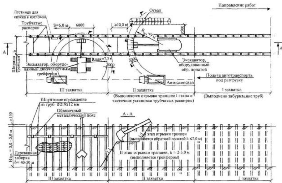
Рисунок 7 - Схема производства работ по разработке грунта траншеи экскаватором и устройства забирок
