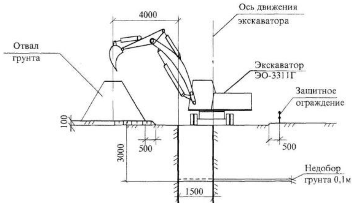
Рисунок 12 - Пример геометрии траншеи для цифровых расчетов
