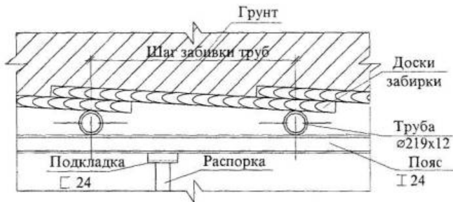
Рисунок 2 - Общая схема траншеи с верхним креплением
