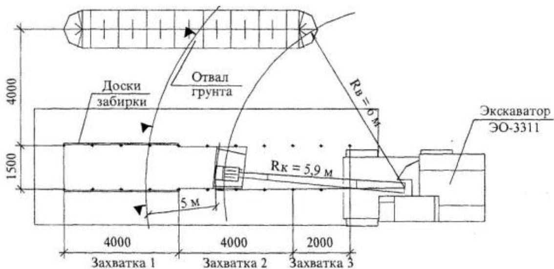
Рисунок 13 - Схемы производства работ по разработке грунта траншеи глубокого заложения с креплением стенок
