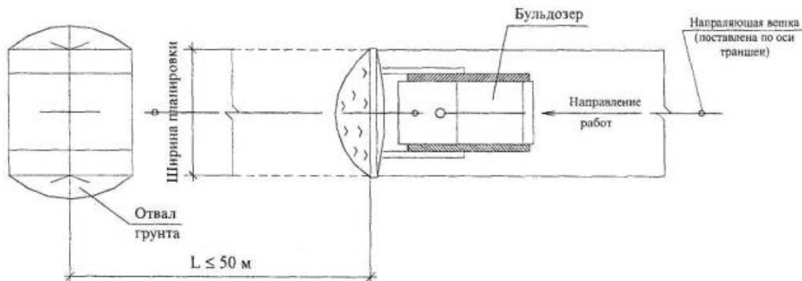
Рисунок 4 - Схема производства работ по планировке поверхности земли бульдозером
