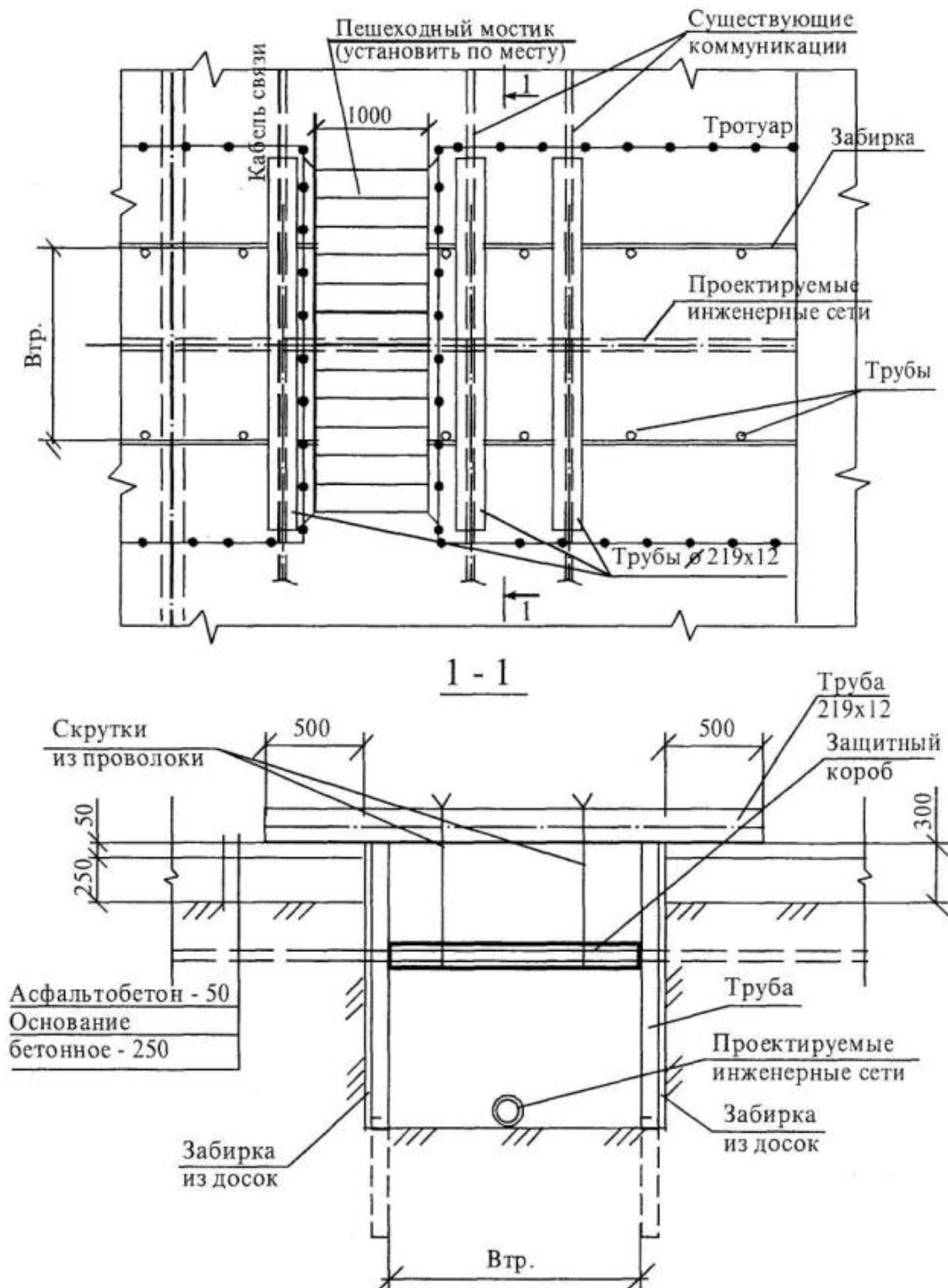
Рисунок 9 - Пример формирования траншеи при пересечении с действующими коммуникациями
