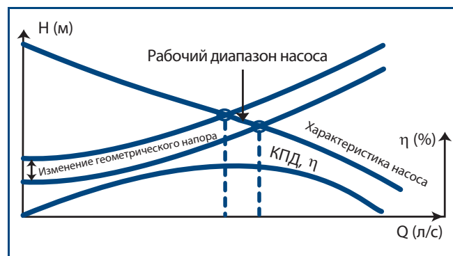
Рис. 23 Рабочая точка для нового насоса и системы с непостоянным геометрическим напором
