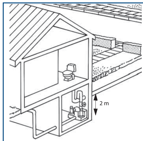
Рис. 88 Схема установки
