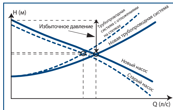
Рис. 24 Смещение рабочей точки с течением времени из-за износа насоса и появления отложений на стенках трубопровода
