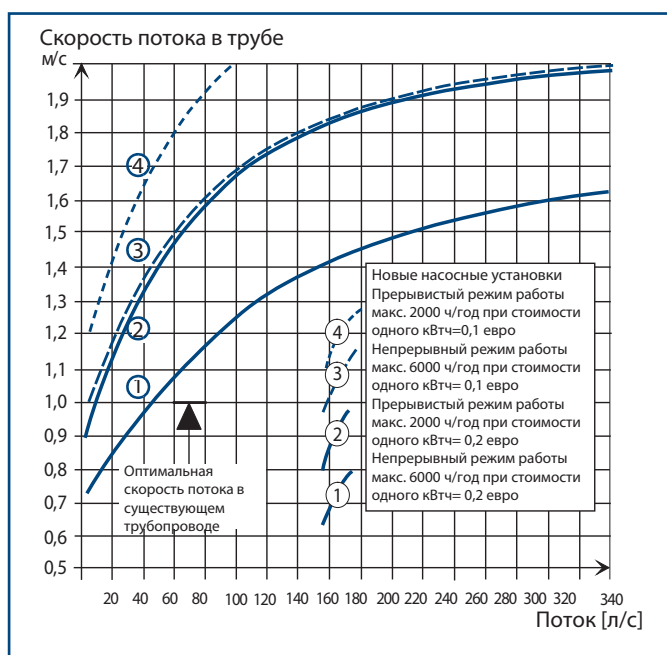
Рис. 71 Определение скорости потока
