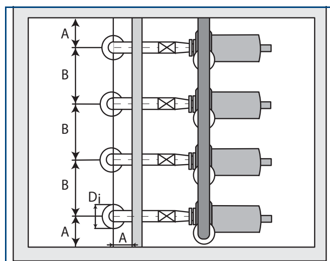
Рис. 63 Рекомендуемые монтажные размеры для установки всасывающих труб в резервуаре насоса ( A_{\text{min}} \geq 1,5 \times D_i и B_{\text{min}} \geq 3 \times D_i )
