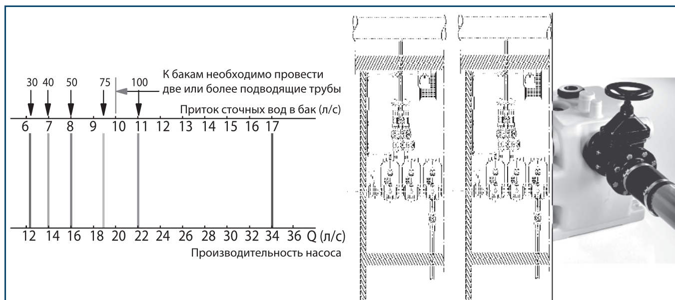
Рис. 59 (Насосная установка MULTILIFT MD 1/MDV : три 400-литровых бака и два насоса с воздушным охлаждением. К бакам требуется подвести две или более подводящие трубы
