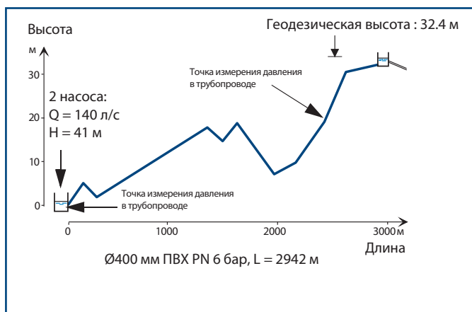
Рис. 73 Продольный профиль напорного трубопровода
