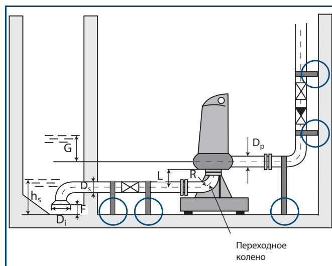
Рис. 61 Рекомендуемые конструктивные размеры всасывающей трубы для вертикального погружного насоса при сухой установке
