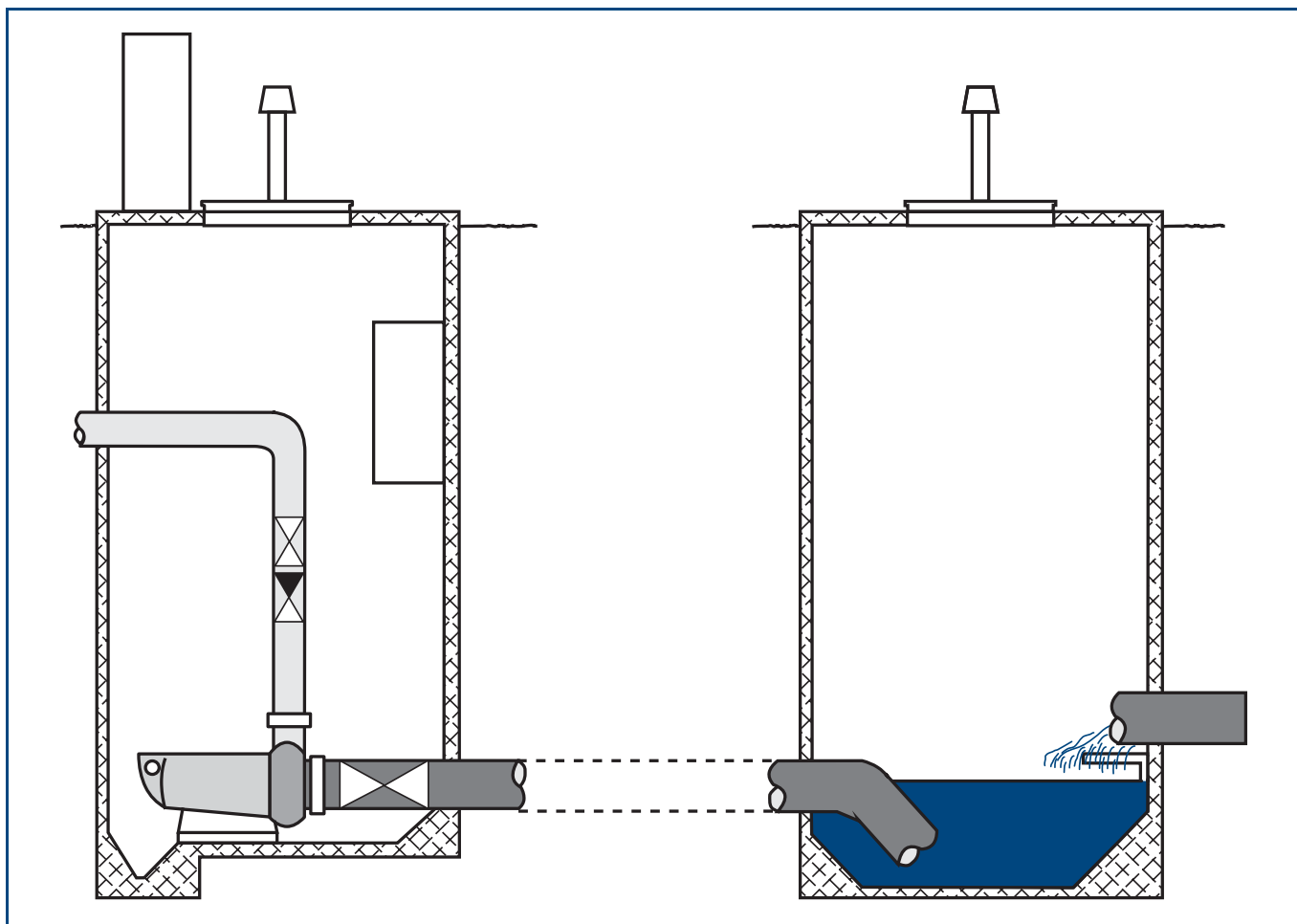
Рис. 51 Если расход входящего потока находится в пределах от 50 л/с до 200 л/с, возможен вариант сухой установки насоса . Этот вариант более затратный, но в случае неисправности насосной установки обеспечивается более быстрый доступ к ней обслуживающего персонала. Это может быть решающим фактором, если вес насоса превышает 100 кг, и для поднятия его на поверхность требуется специальное оборудование.
