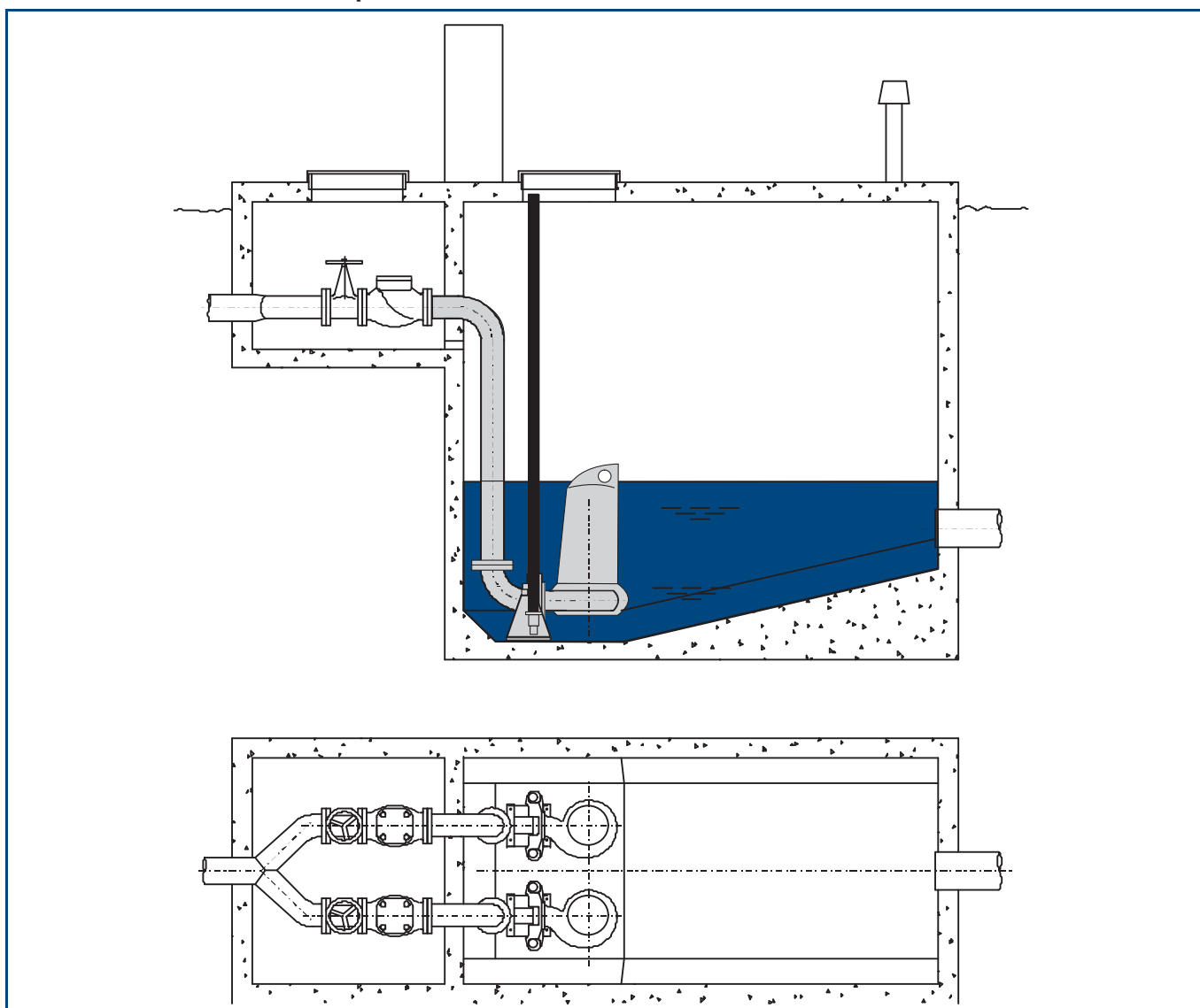
Рис. 52 Если максимальный расход входящего потока превышает 200 л/с, можно рассмотреть вариант резервуара, дно которого находится под наклоном и имеет удлиненную форму, за счет чего происходит гашение энергии жидкости, поступающей в резервуар. Также предотвращается появление турбулентных завихрений и частая замена бетонной плиты наряду с другим оборудованием. Перед всасывающим патрубком насоса, на горизонтальной поверхности дна резервуара часто требуется установка устройства для гашения волн
