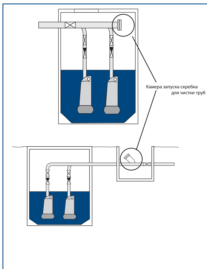
Рис. 72 Камера запуска скребка для чистки труб
