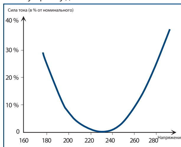
Рис. 42 Увеличение энергопотребления в зависимости от напряжения питания
