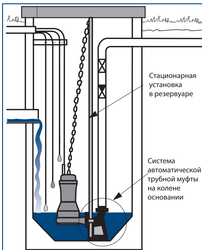
Рис. 28 Старайтесь избегать такой конструкции для перекачки высокорррозионных жидкостей. Поскольку трубные соединения погружены в жидкость, обнаружить протечки и разведенный в результате коррозии металл при внешнем осмотре оборудования будет невозможно.
