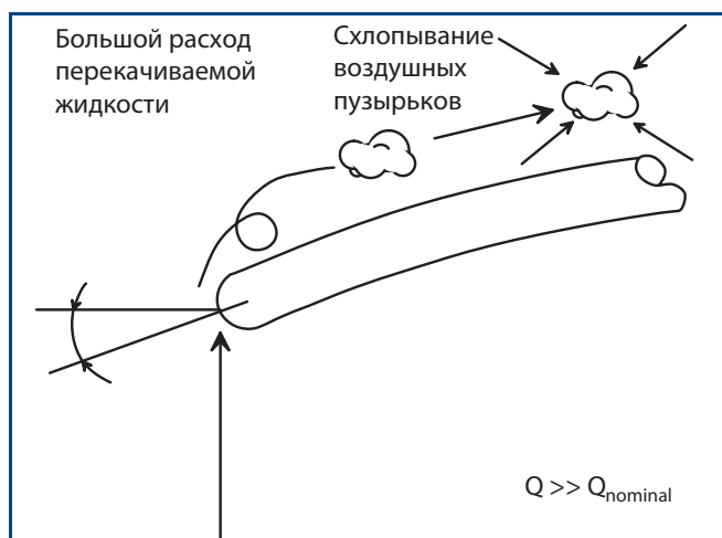
Рис. 29 Перекачиваемая жидкость ударяется о входную кромку лопасти рабочего колеса под углом отличным от угла лопатки. Вихри и зоны пониженного давления образуются на обратной стороне рабочего колеса. Если давление становится ниже давления насыщенного пара, то возникают пузырьки пара. Переместившись совместно с потоком в зону повышенного давления, они неизбежно взорвутся. Это может привести к образованию раковин и коррозии на поверхности, расположенной рядом с областью повышенного давления.
