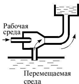
Рис. 1.8. Струйный насос
