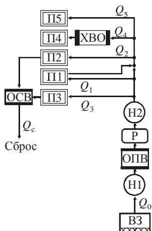
Рис. 7.2. Последовательная каскадная система водоснабжения
