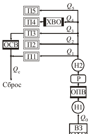
Рис. 7.1. Прямоточная система водоснабжения
