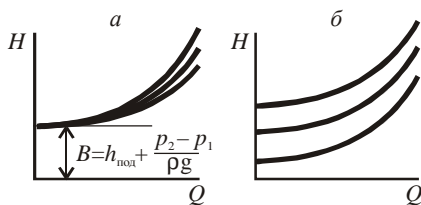
Рис. 2.2. Изменение напорной характеристики сети: а – при изменении коэффициента местного сопротивления; б – при изменении давления в точке нагнетания
