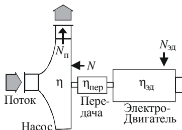
Рис. 1.12. Потери энергии в насосной (вентиляторной) установке
