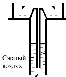
Рис. 1.9. Эрлифт
