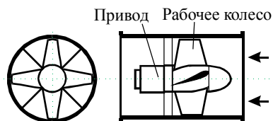
Рис. 1.3. Осевой нагнетатель
