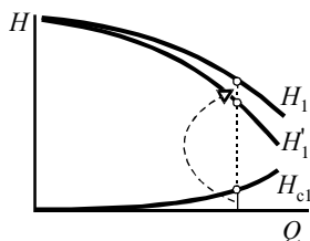
Рис. 3.14. Сопротивление участка подсоединения H_{cl} и напорная характеристика H'_1 , отнесенная к точке присоединения нагнетателя к сети
