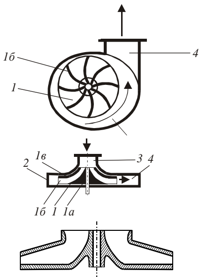
Рис. 4.1. Центробежный нагнетатель:
