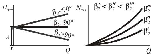
Рис. 4.7. Теоретические характеристики центробежных нагнетателей
