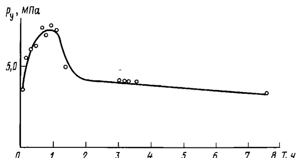
Рис. 9.10. Изменение устьевое давления при освоении скв. 534 Битковского месторождения азотом (закачка в лифт)
