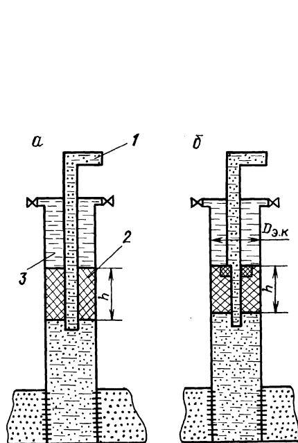
Рис. 7.6. Технологические схемы пакерования скважин ОК (а) и СКУ (б): 1 – шток ( \rho \geq 1120 \text{ кг/м}^3 ); 2 – ППЖ; 3 – пресная или пластовая вода ( \rho \leq 1300 \text{ кг/м}^3 ); h – высота пакера из ППЖ
