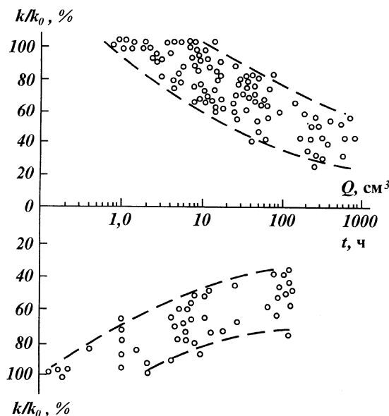
Рис. 4.2. Зависимость степени снижения проницаемости в зоне кольтатации k/k_0 от объема промывочной жидкости Q , проникшей в пласт, и времени фильтрации t
