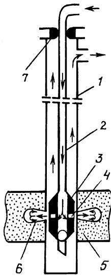
Рис. 6.11. Схема перфорации в скважине гидropескоструйным методом: 1 - обсадная колонна; 2 - НКТ; 3 - АП; 4 - насадка; 5 - пласт; 6 - каналы ГПП; 7 - сальник
