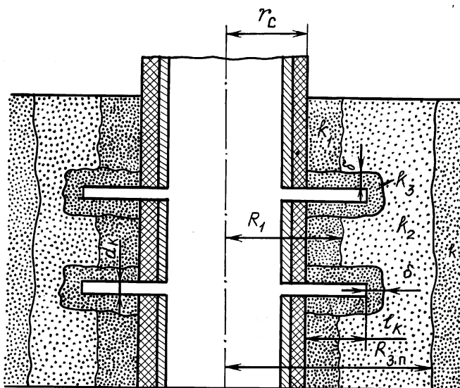
Рис. 3.7. Схематическое изображение призабойной зоны и забоя перфорированной скважины:
