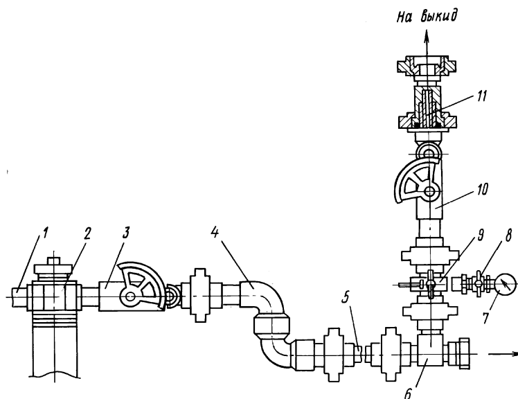
Рис. 2.17. Упрощенная схема обвязки устья скважины:
