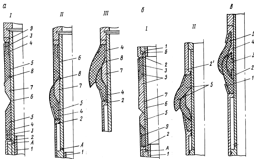
Рис. 1.3. Секционные уплотняющие элементы гидромеханического пакера: a, б – первый и второй основные элементы; в – дополнительный элемент
