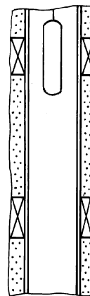
Рис. 1.7. Схема установки взрывных пакеров
