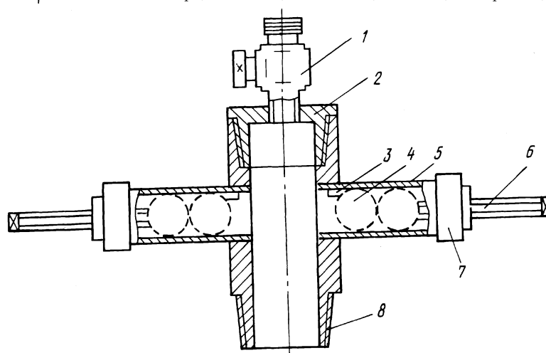
Рис. 7.3. Цементирующая головка кассетного типа:
