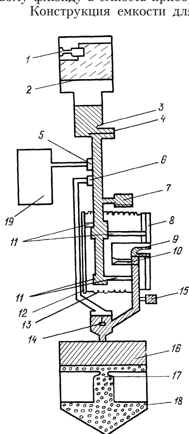
Рис. 2.19. Принципиальная схема испытателя пластов на кабеле фирмы "Шлюмберже"
