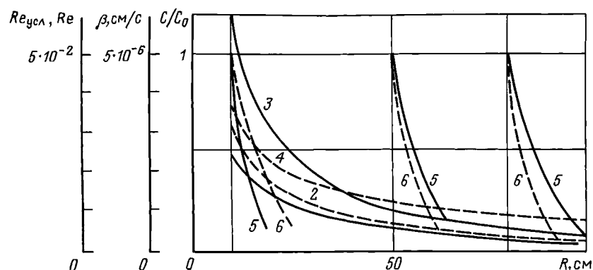
Рис. 9.15. Изменение гидродинамических условий Re_{усл} (1), Re (2), коэффициента массопередачи \beta (3, 4) и профилей нейтрализации C/C_0 плавиковой кислоты (5, 6) при ее радиальном распространении: 1, 3, 5 – негазированная глинокислота ( \Gamma_p = 0 ); 2, 4, 6 – газированная глинокислота ( \Gamma_p = 1,5 )
