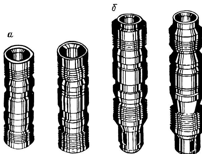
Рис. 5.13. Пакеры взрывные: шлицовый (а) и цементировочный (б)
