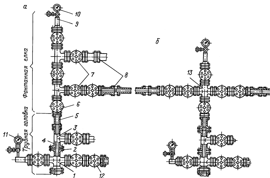
Рис. 5.3. Фонтанная арматура:
