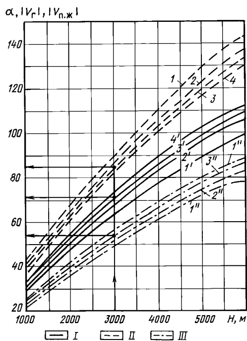
Рис. 9.7. Номограмма для расчета процесса вызова притока из пласта пеной с самоизливом и последующим осушением скважины газообразным азотом:
