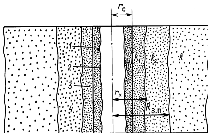
Рис. 3.2. Схема призабойной зоны после вскрытия продуктивного пласта бурением: 1 – стенка скважины; 2 – глинистая корка; 3 – зона коагуляции; 4 – зона проникновения фильтрата бурового раствора; k , k_1 , k_2 – проницаемость соответственно природная, в зоне коагуляции и в зоне проникновения фильтрата
