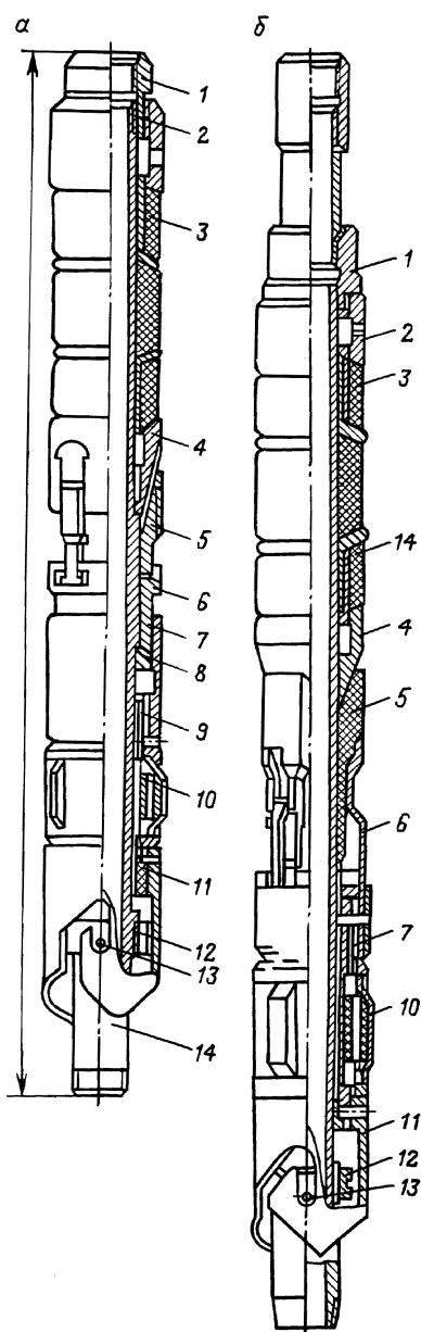
Рис. 5.5. Пакер ПН-ЯМ с внешним диаметром 150, 160, 185, 210, 236, 265 мм (≠) и 118, 136 мм (•): 1 – головка; 2 – упор; 3 – манжеты; 4 – конус; 5 – плашка; 6 – плашкодержатель; 7 – цилиндр; 8 – захват; 9 – корпус фонаря; 10 – башмак; 11 – замок; 12 – гайка; 13 – палец; 14 – ствол
