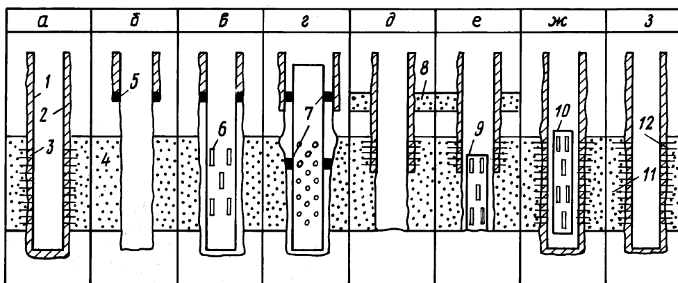
Рис. 1.1. Основные типы забоев скважин:
