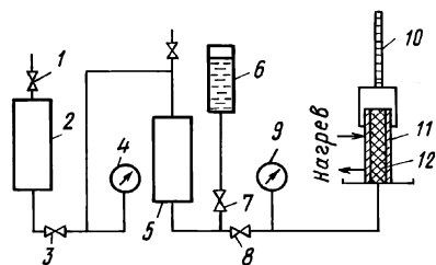
Рис. 7.12. Пластомер:
