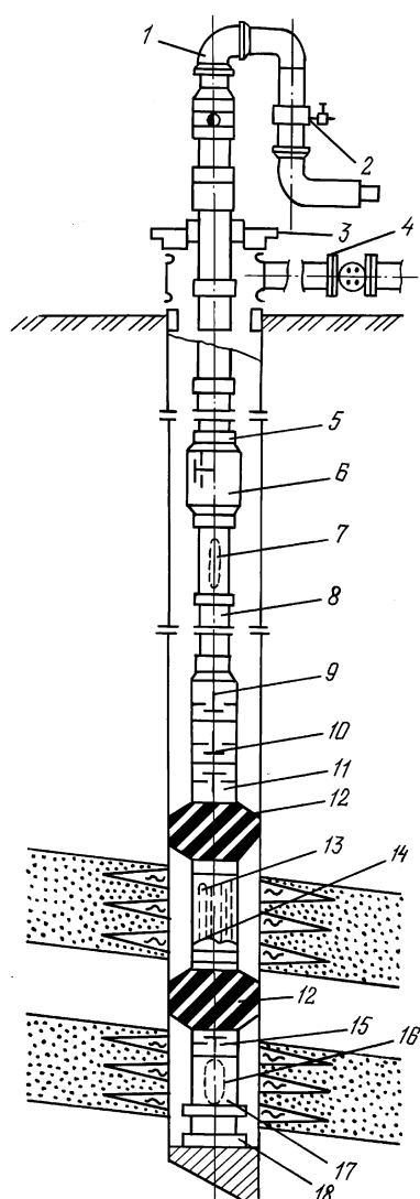
Рис. 2.3. Схема компоновки испытателя пластов с двумя пакерами и с упором "ноги" на забой скважины: 1 — быстросъемные трубы; 2 — пробный кран; 3 — стол ротора; 4 — задвижка превентора; 5 — колонна бурильных труб; 6 — циркуляционный клапан; 7 — верхний манометр; 8 — бурильная труба; 9 — запорно-поворотный двухцикловой клапан; 10 — испытатель пластов; 11 — ясс; 12 — пакер ПЦ; 13 — основной манометр для записи КВД; 14 — щелевой фильтр; 15 — уравнильный клапан; 16 — контрольный манометр; 17 — утяжеленные бурильные трубы; 18 — упорный башмак
