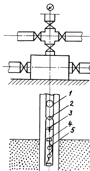
Рис. 6.5. Схема выполнения работ перфоратором, спускаемым по трубам (типа ПНК): 1 — резиновый шар; 2 — циркуляционный клапан; 3 — ударно-накольный механизм; 4 — приспособление иницирования зарядов; 5 — перфоратор
