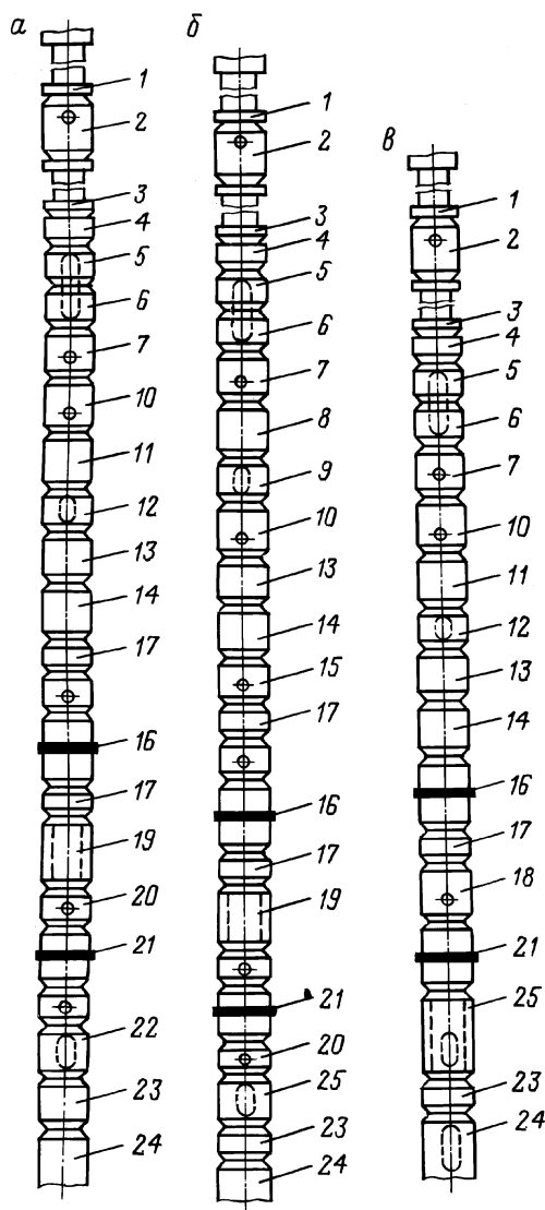
Рис. 2.6. Компоновка испытателей пластов: a – с двумя пакерами; б – селективного испытания объектов; в – многоциклового испытания объектов в наклонно направленных стволах; 1, 3 – бурильные трубы; 2 – циркуляционный клапан; 4, 17, 23 – переводники; 5, 6, 9, 12, 25 – патрубки; 7 – штуцер; 8 – запорно-поворотный клапан; 10 – ИИП; 11 – приспособление для вращения; 13 – пробоотборник; 14 – ясс; 15 – безопасный замок; 16, 21 – пакер; 18 – распределяющее приспособление; 19 – фильтр; 20 – уравнительное приспособление; 22 – фильтр; 24 – хвостовик
