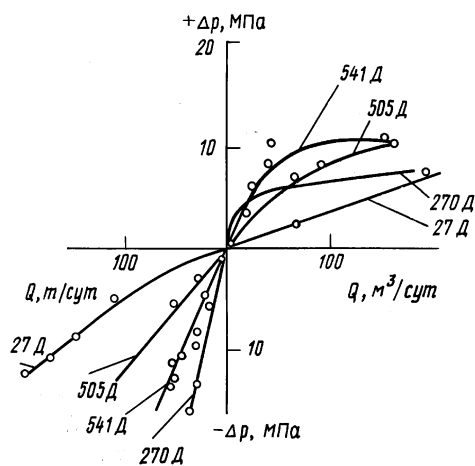
Рис. 11.2. Индикаторные кривые скважин Долинского месторождения, снятые при отборе и нагнетании: Q , т/сут – дебит при эксплуатации; Q , м³/сут – приемистость при нагнетании; +\Delta p – репрессия на пласт; -\Delta p – депрессия на пласт. Цифры у кривых – номера скважин
