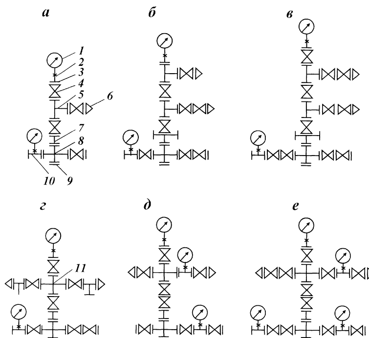
Рис. 5.4. Типовые схемы оборудования устья скважины:
