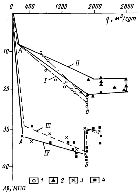
Рис. 11.4. Индикаторные кривые ГРП: I, II – скв. 505 Д; III – скв. 549 Д; IV – скв. 282 Д; 1, 2, 3, 4 – режимы, при которых производилась закачка песка в пласт; \Delta p – репрессия на пласт при ГРП; q – расход жидкости
