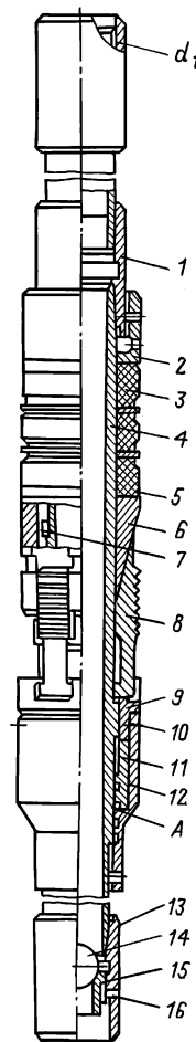
Рис. 5.6. Пакер ПН-ЯГМ: 1 – муфта; 2 – упор; 3 – манжета; 4 – ствол; 5 – обойма; 6 – корпус; 7 – шпонка; 8 – плашка; 9 – плашкодержатель; 10 – винт; 11 – кожух; 12 – поршень; 13 – корпус клапана; 14 – шарик; 15 – седло; 16 – срезной винт
