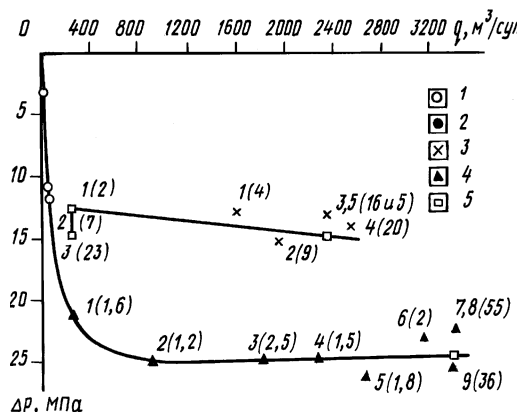
Рис. 11.7. Индикаторные кривые при закачке жидкости в скв. 57 Д:
