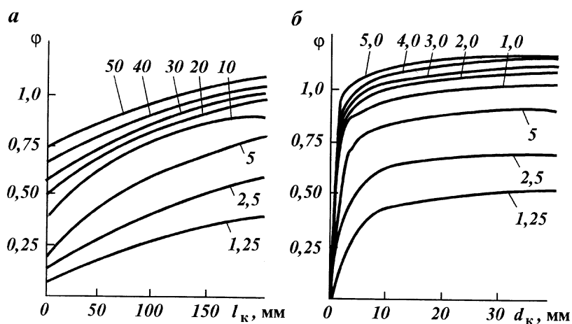
Рис. 3.5. Зависимость коэффициента гидродинамического совершенства скважины от параметров перфорации ( R_k = 400 м; r_c = 0,1 м): а – от длины канала перфорации; d_k = 12 мм; б – от диаметра канала перфорации; l_k = 150 мм; цифры на кривых – плотность перфорации, отверстие на 1 м
