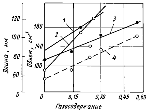
Рис. 9.25. Влияние газосодержания на длину (1, 3) и объем (2, 4) перфорационных каналов: 1, 2 – для образцов с \sigma_{сж} = 39 МПа, \Delta p = 11 МПа, d_n = 6 мм; 3, 4 – для образцов с \sigma_{сж} = 60 МПа, \Delta p = 20 МПа, d_n = 4,5 мм
