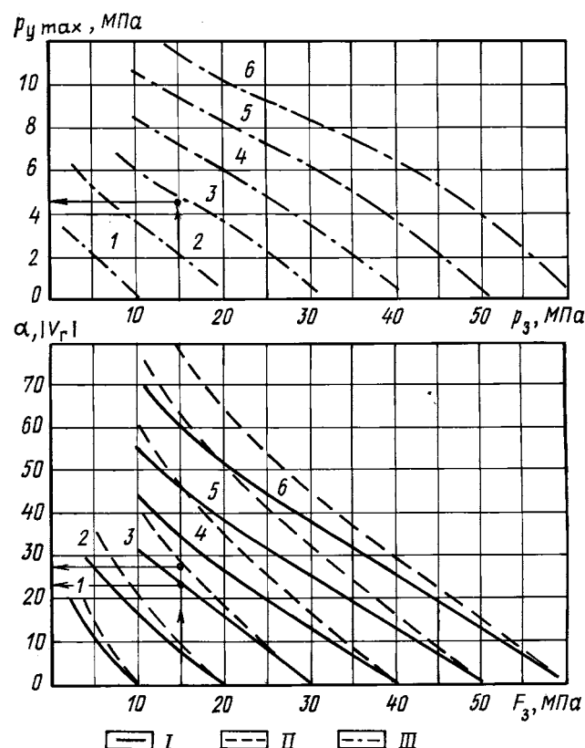
Рис. 9.6. Номограммы для расчета процесса вызова притока из пласта с применением пены с последующим ее самоизливом из скважины ( \rho_{\text{ж}} = 1000 \text{ кг/м}^3 ): I – относительный объем газа |V_r| ; II – степень газификации \alpha ; III – максимальное устьевое давление p_{y \max} ; 1, 2, 3, 4, 5, 6 – глубина осваиваемой скважины соответственно 1000, 2000, 3000, 4000, 5000, 6000 м; p_z – забойное давление; \alpha , |V_r| – безразмерные величины
