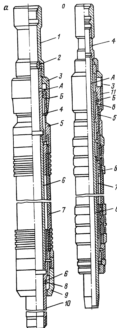
Рис. 5.10. Рукавный пакер типов ПД-Г (⊗) и ПД-Г (·): 1 – патрубок; 2 – седло; 3 – поршень; 4 – переводник; 5 – головка; 6 – ствол; 7 – рукав; 8 – манжета; 9 – ниппель; 10 – хвостовик; 11 – уплотняющее кольцо
