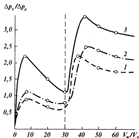
Рис. 6.8. Характер изменения \Delta p_t/\Delta p_0 при использовании солевых растворов: 1 – 10 %-ный раствор KCl; 2 – 0,3 %-ный раствор ПАВ + 20 %-ный раствор CaCl 2 ; 3 – ИЭР
