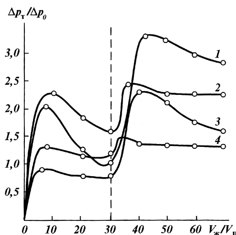
Рис. 6.7. Характер изменения \Delta p_t/\Delta p_0 при двухфазной фильтрации в пласт
