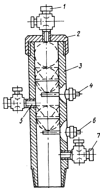
Рис. 7.2. Цементирующая головка:
