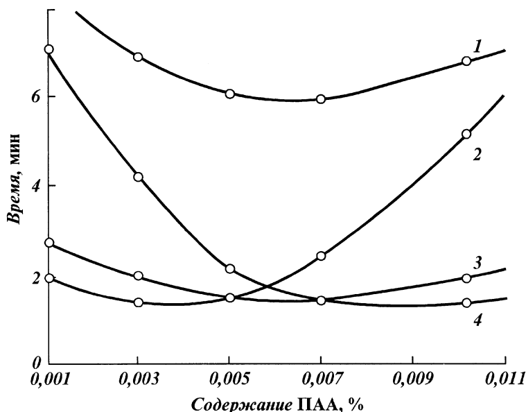
Рис. 6.9. Характер флокуляции частиц при различном содержании полимеров: 1 – 10 %-ный раствор NaCl, C_t = 2000 мг/л; 2 – 10 %-ный раствор \text{CaCl}_2 , C_t = 500 мг/л; 3 – 10 %-ный раствор \text{CaCl}_2 , C_t = 2000 мг/л; 4 – 10 %-ный раствор \text{CaCl}_2 , C_t = 5000 мг/л
