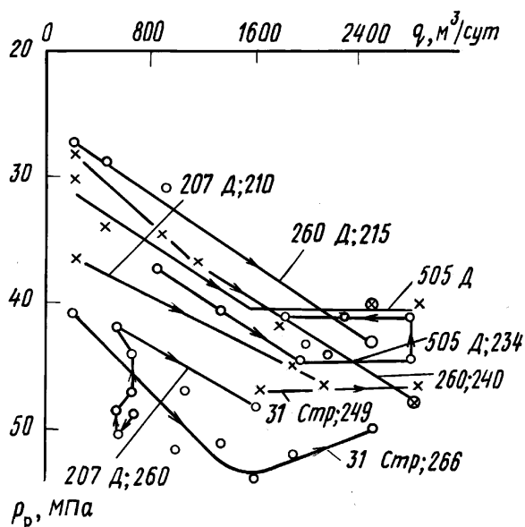
Рис. 11.5. Индикаторные кривые повторных ГРП при изменении пластового давления:
