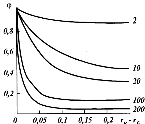
Рис. 3.3. Влияние параметров зоны кольтации на коэффициент гидродинамического совершенства скважины при \beta_1 = 1 . Шифр кривых – степень снижения проницаемости \beta_2
