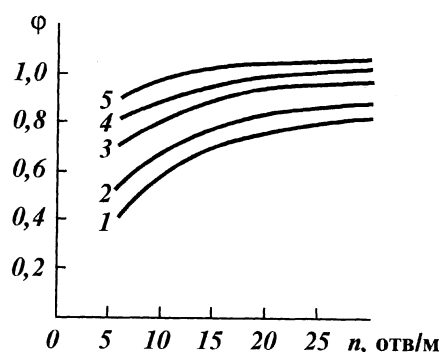
Рис. 3.6. Зависимость коэффициента гидродинамического совершенства скважины от плотности перфорации ( R_k = 450 м, r_c = 0,1 м; d_k = 12 мм): 1, 2, 3, 4, 5 – l_k соответственно 25, 50, 100, 150 и 200 мм
