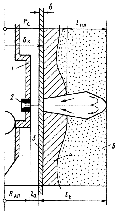
Рис. 6.13. Схема формирования канала ГПП в скважине: 1 - гидropескоструйный аппарат; 2 - насадка; 3 - колонна; 4 - цементное кольцо; 5 - пласт
