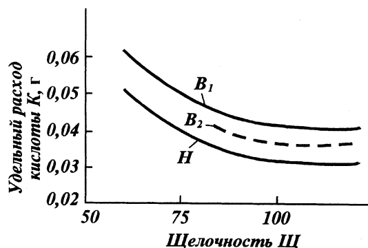
Рис. 7.9. Зависимость количества добавляемой кислоты \bar{a} от щелочности \bar{b} гипана
