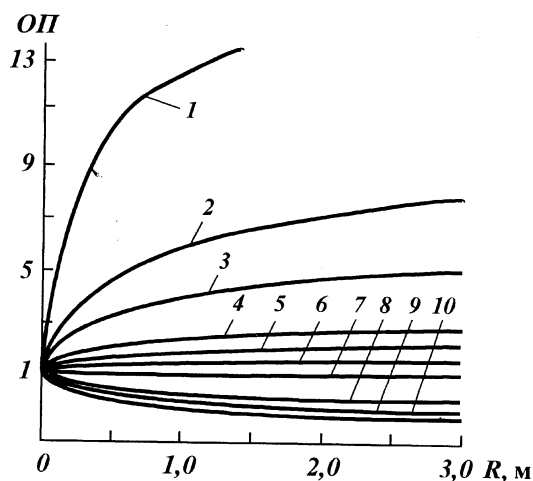
Рис. 4.1. Зависимость снижения продуктивности скважин от радиуса и степени снижения проницаемости k/k_0 в околоскважинной зоне:
