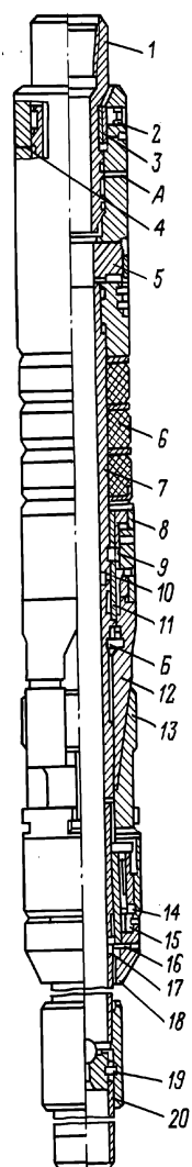
Рис. 5.9. Пакер ПД-ЯГМ: 1 – шток; 2 – специальный винт; 3, 4, 8, 15, 16, 19 – срезные винты; 5, 13 – верхняя и нижняя плашки; 6 – манжета; 7 – ствол; 9 – захват; 10, 14 – штипы; 11 – поршень; 12 – корпус; 17 – втулка; 18 – центратор; 20 – седло
