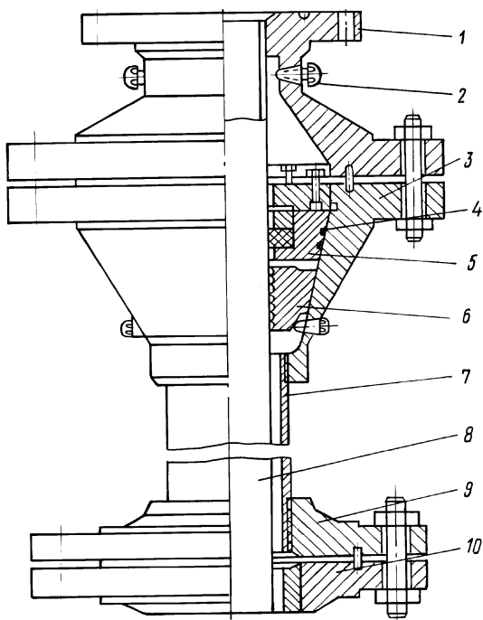
Рис. 5.1. Колонная головка клиновая типа ГКК:
