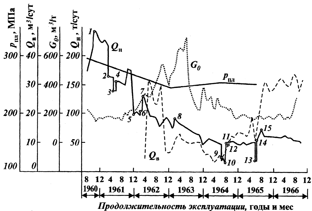
Рис. 4.6. Изменение среднесуточной производительности скв. 222 во времени:
