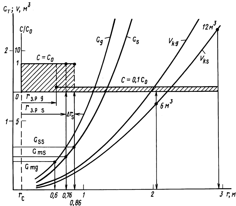
Рис. 10.6. Развитие зоны растворения пласта во время ГКО и профиль нейтрализации кислоты (типичная картина):
