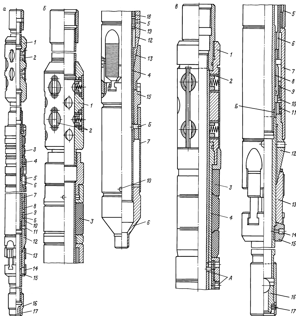
Рис. 5.7. Пакер ПД-ЯГ:
