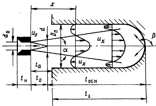
Рис. 6.12. Схема вытекания потока в канал
