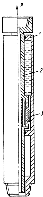
Рис. 2.10. Ясс закрытого типа
