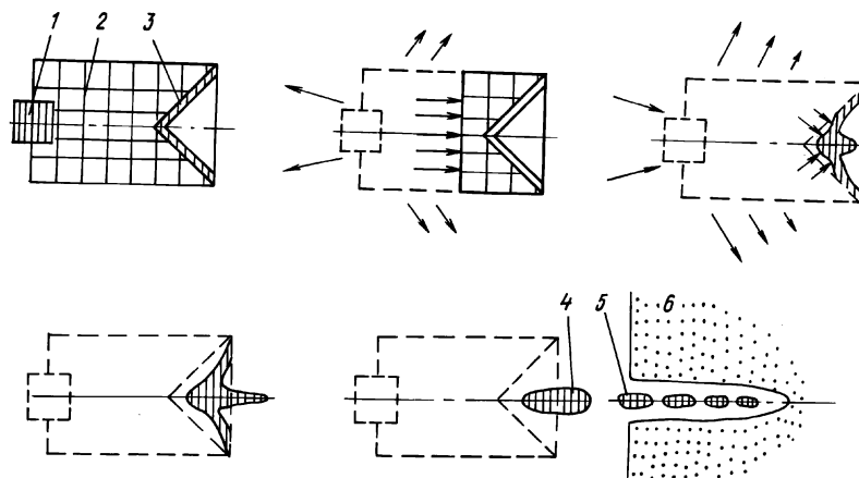
Рис. 6.1. Схема распределения кумулятивной струи:
