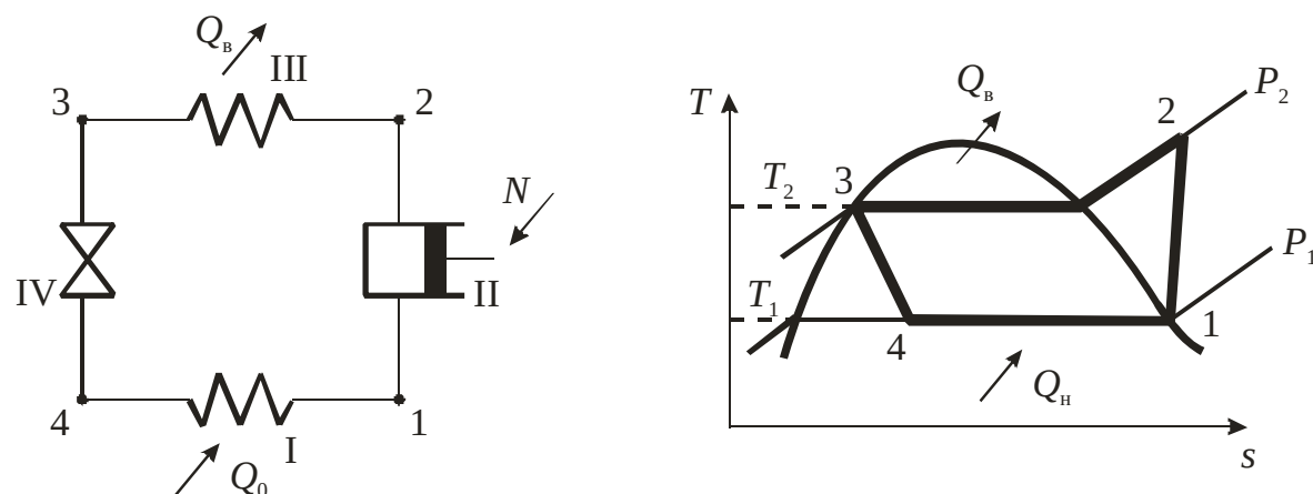
Рис.23. Схема парокомпрессионного теплового насоса и его цикл в T-s – диаграмме. I – испаритель, II – компрессор, III – конденсатор, IV – дроссель.
