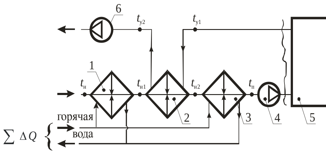
Рис. 4.3. Принципиальная схема системы вентиляции с теплообменником-утилизатором. 1 – предварительный подогреватель (калорифер), 2 – рекуперативный теплообменник, 3 – подогреватель (калорифер), 4 – приточный вентилятор, 5 – вентилируемое помещение,
