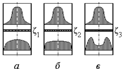
Рис.11. Изменение неравномерного профиля скорости рабочей среды на тонком аэродинамическом сопротивлении (коэффициент гидродинамического сопротивления \zeta_1 < \zeta_2 < \zeta_3 , \zeta_2 = \zeta_{\text{орт}} ).
