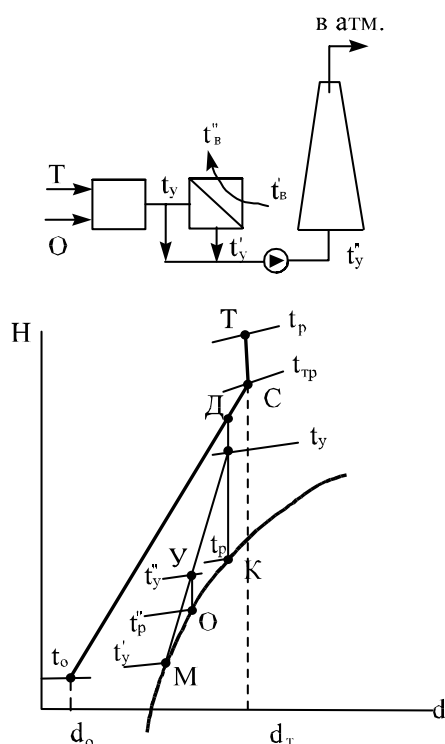
Рис. 6. Принципиальная схема байпасирования уходящих газов и изображение изменения их состояния в H-d- диаграмме
