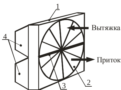
Рис.22. Схема регенеративного теплообменника с вращающейся насадкой.
