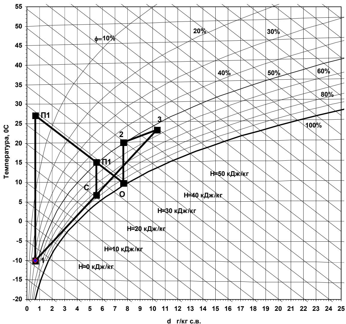
Рис. 4.2 Изменение состояния влажного воздуха в системе кондиционирования общественного здания.
