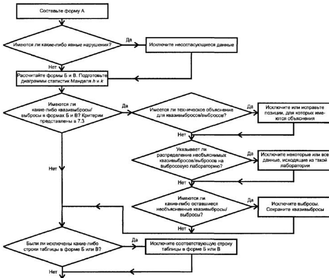
Рисунок 3 - Структурная схема принципиальных этапов статистического анализа (см. продолжение)
