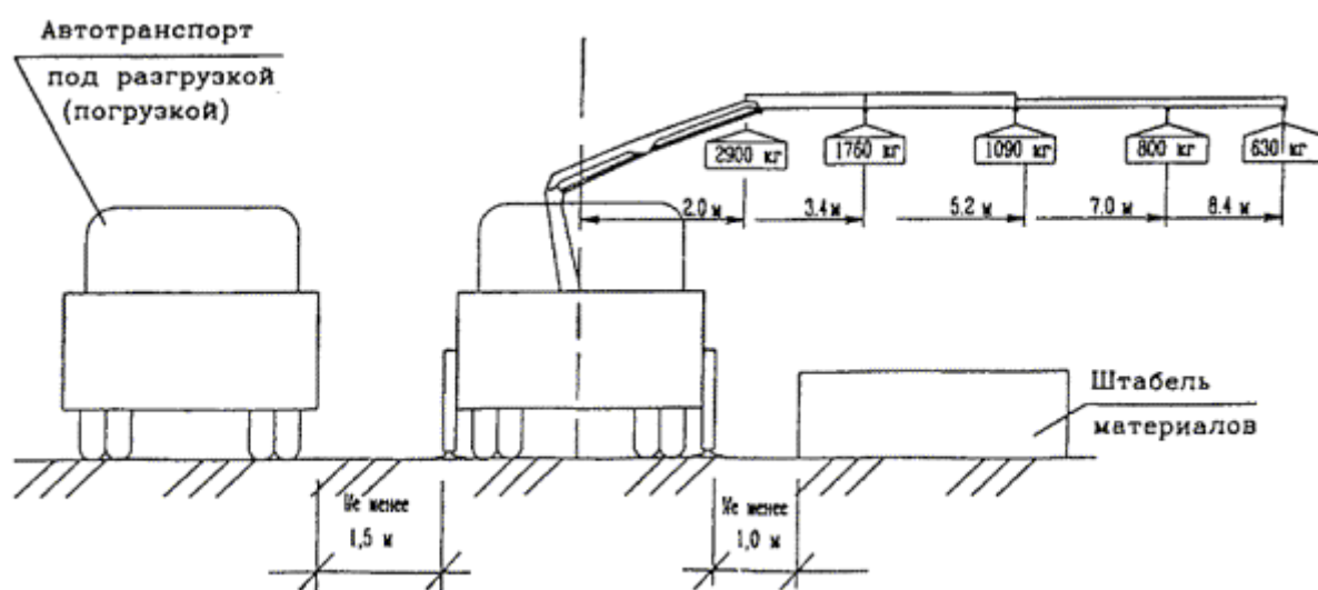
Рисунок 3 - Вертикальная привязка крана-манипулятора ПК 7000
