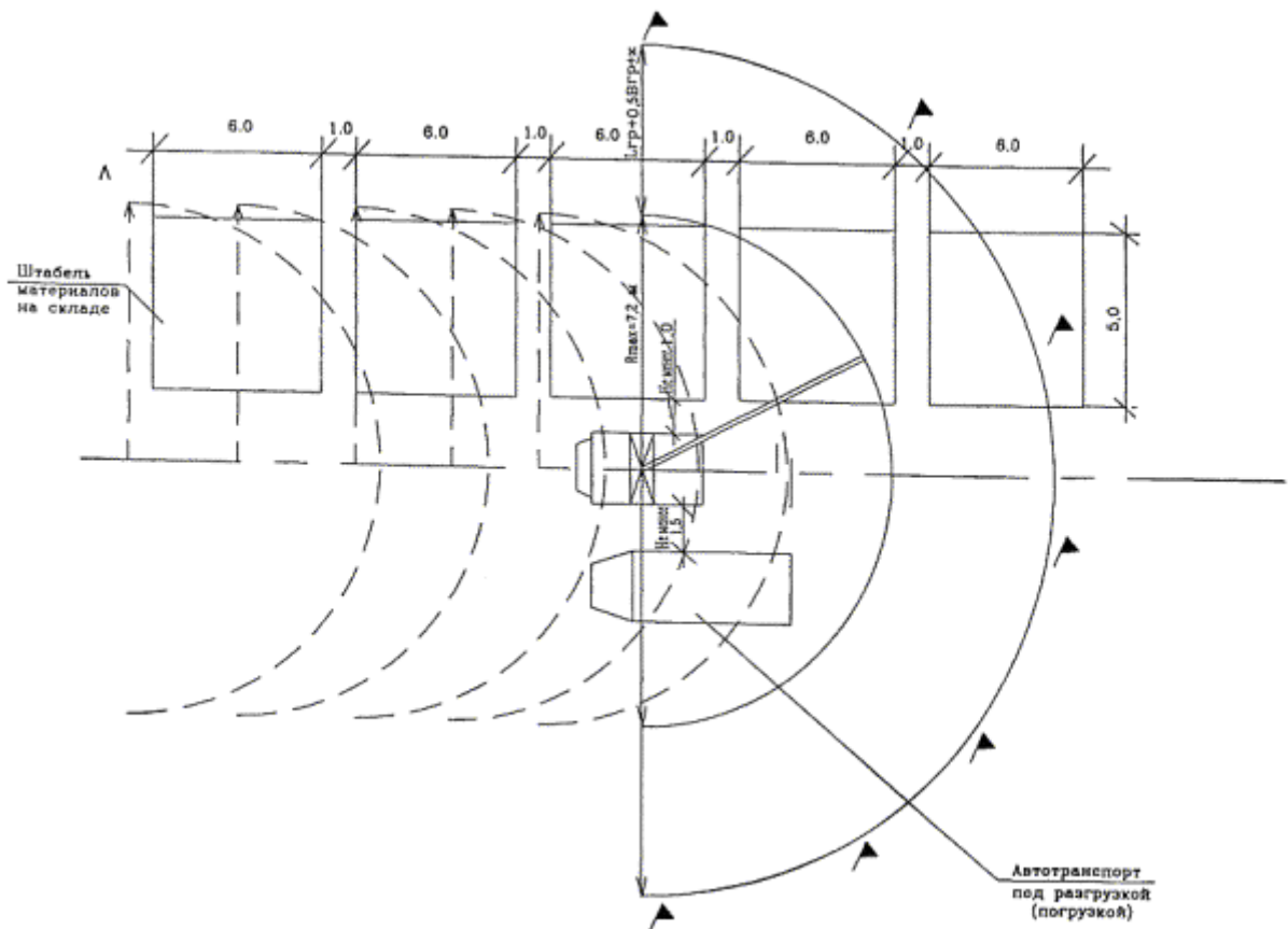
Рисунок 8 - Горизонтальная привязка крана-манипулятора ПКК 8000
