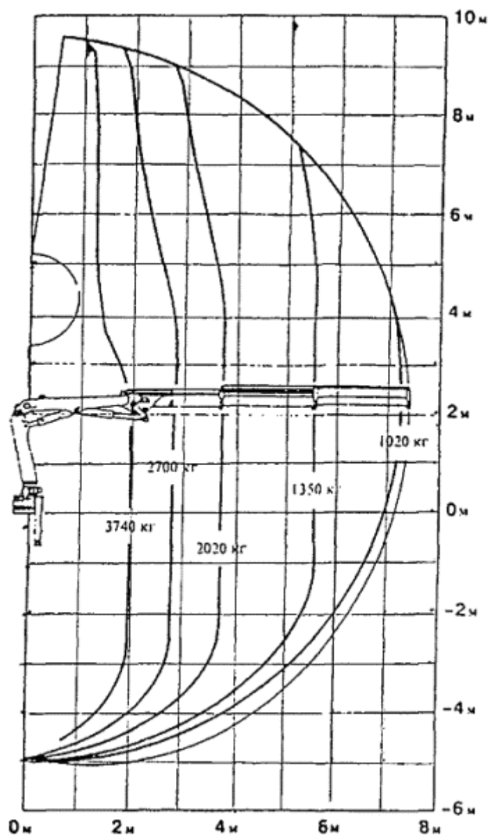
Рисунок 6 - Диаграмма грузоподъемности крана-манипулятора ПКК 8000
