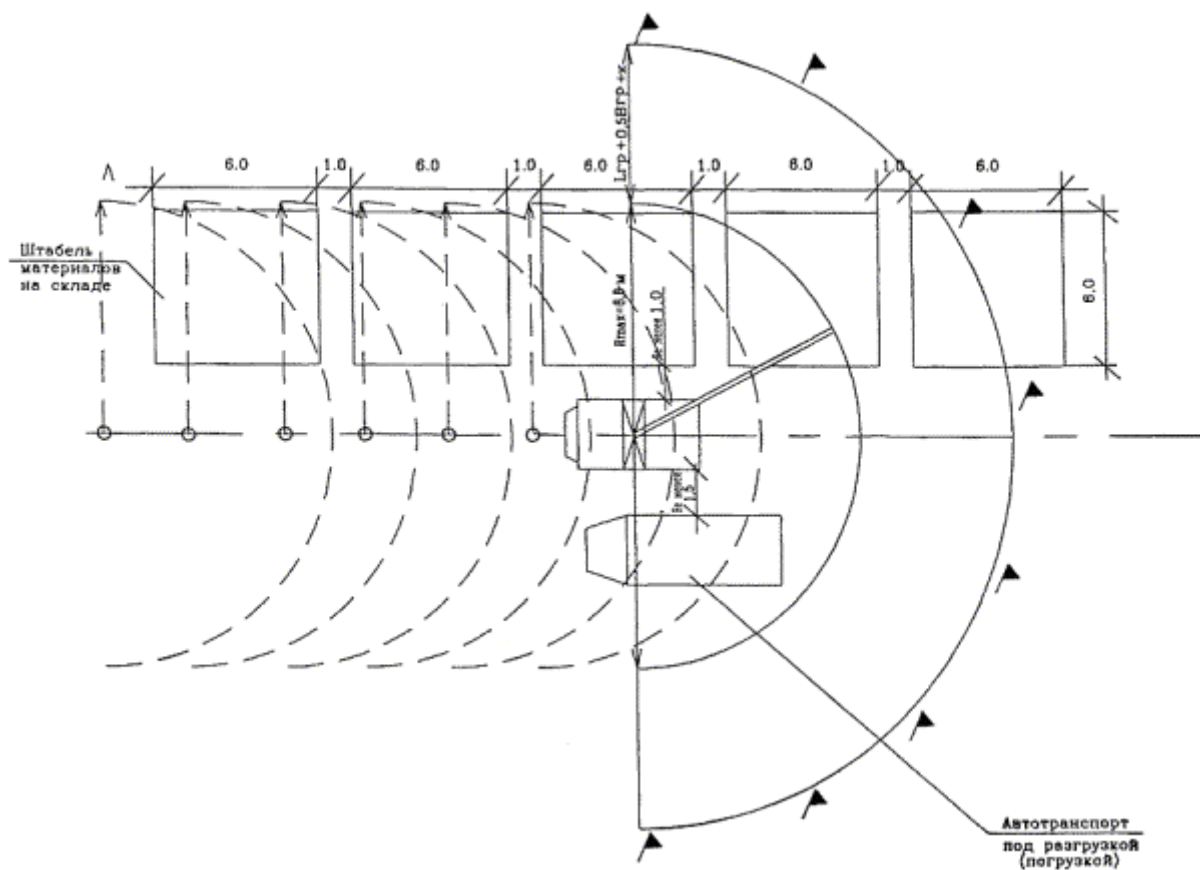
Рисунок 4 - Горизонтальная привязка крана-манипулятора ПК 7000
