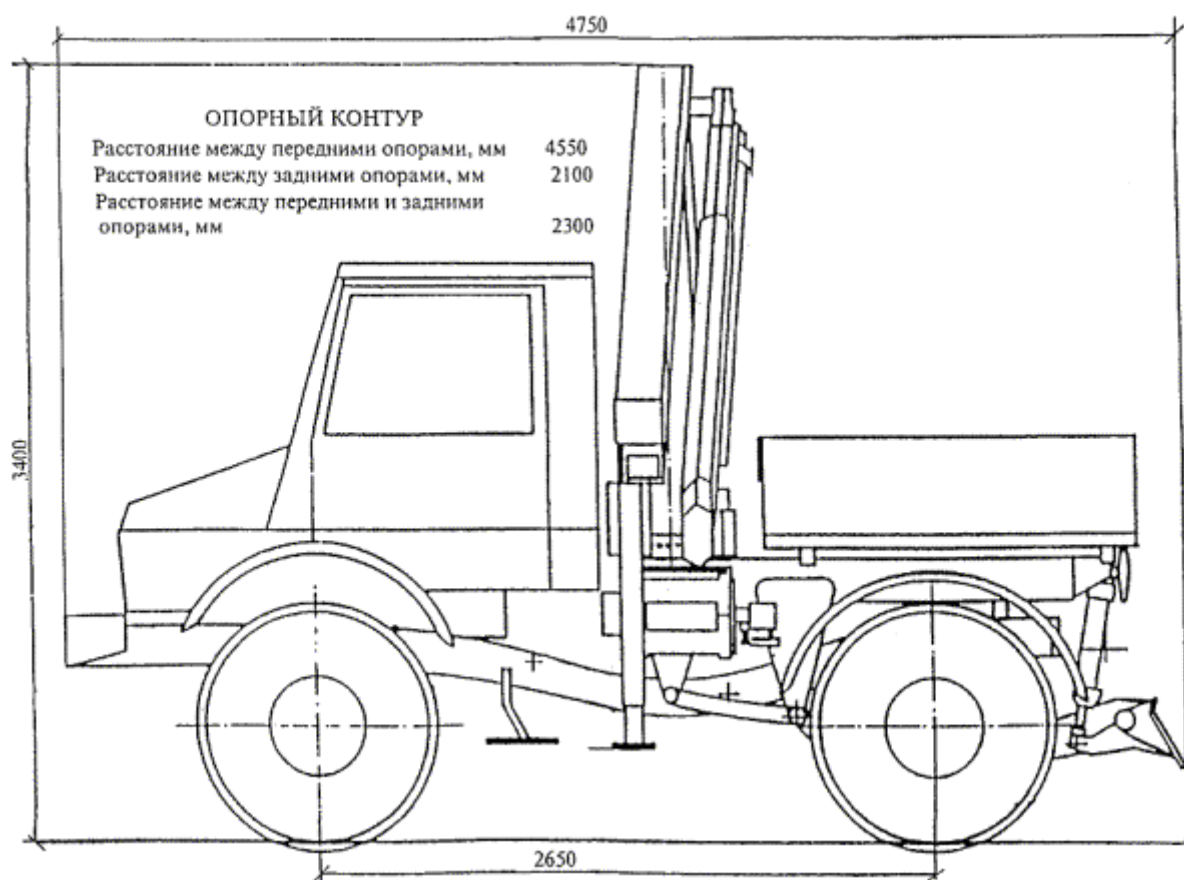
Рисунок 5 - Общий вид крана-манипулятора ПКК 8000
