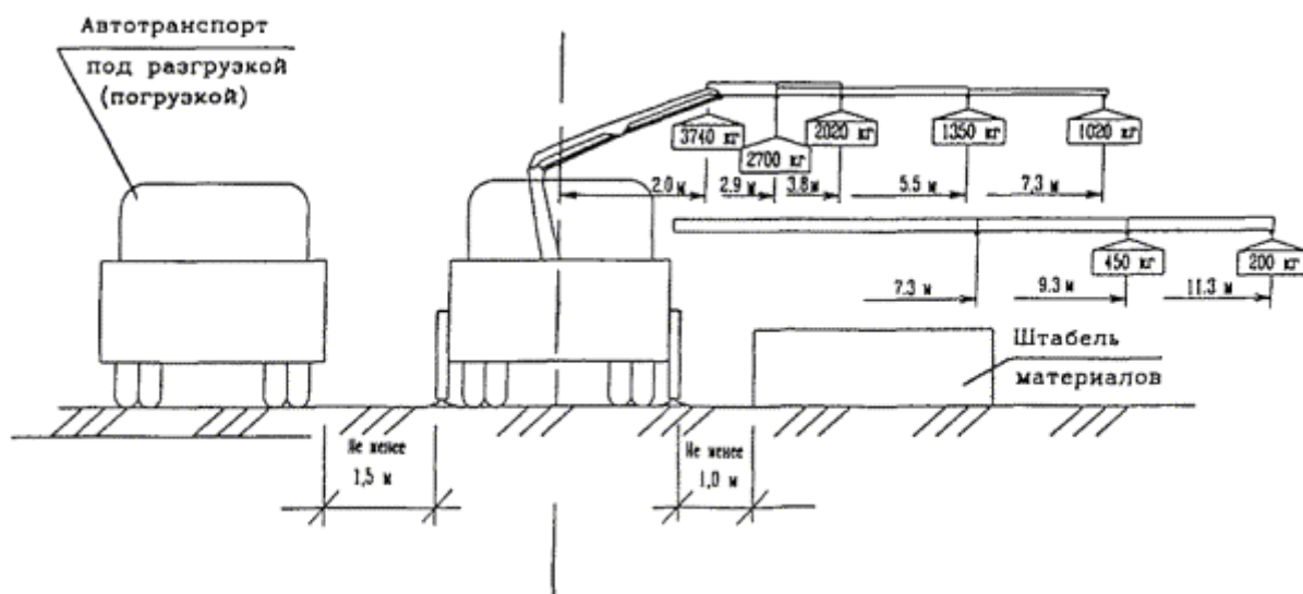
Рисунок 7 - Вертикальная привязка крана-манипулятора ПКК 8000
