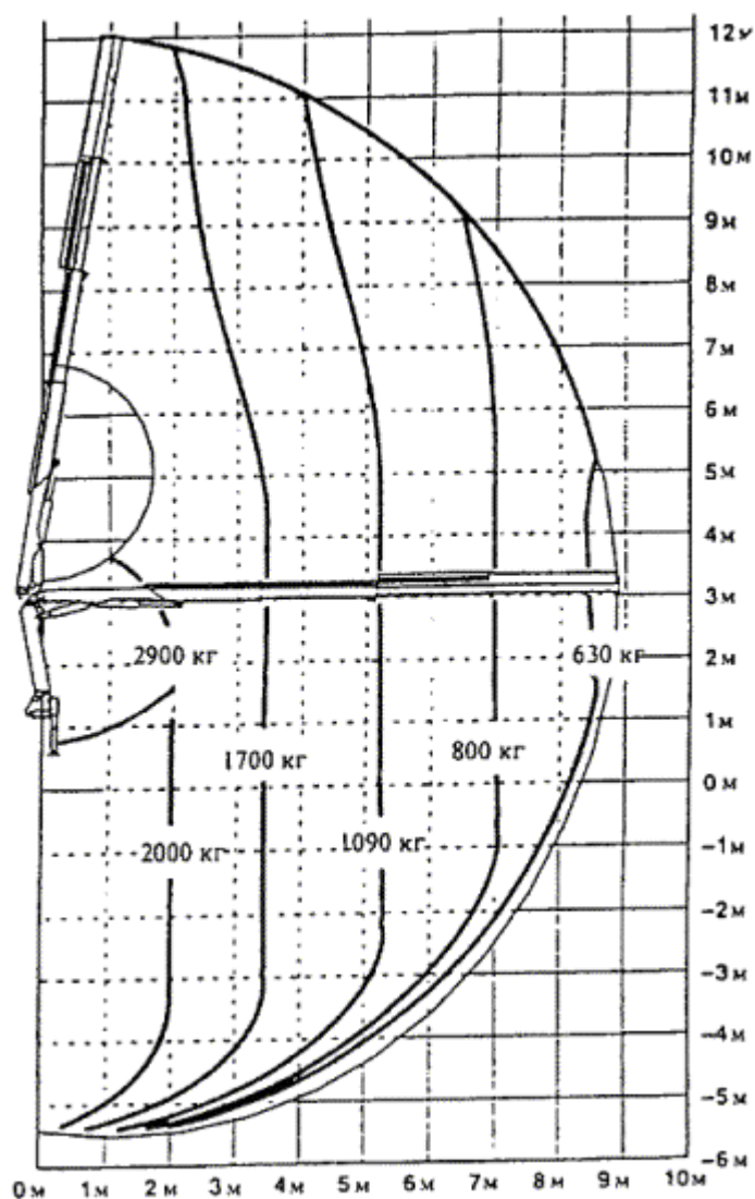
Рисунок 2 - Диаграмма грузоподъемности крана-манипулятора ПК 7000
