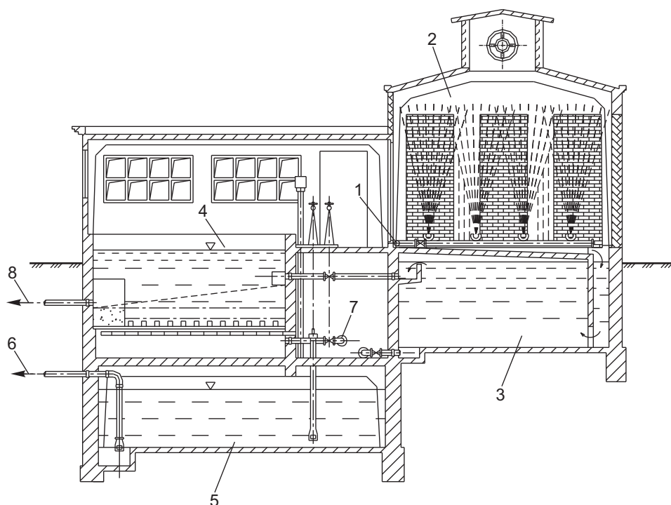
1 — подача исходной воды; 2 — аэрационный зал; 3 — отстойник; 4 — скорый фильтр; 5 — РЧВ; 6 — отвод чистой воды; 7 — подача воды на промывку; 8 — отвод воды после промывки
