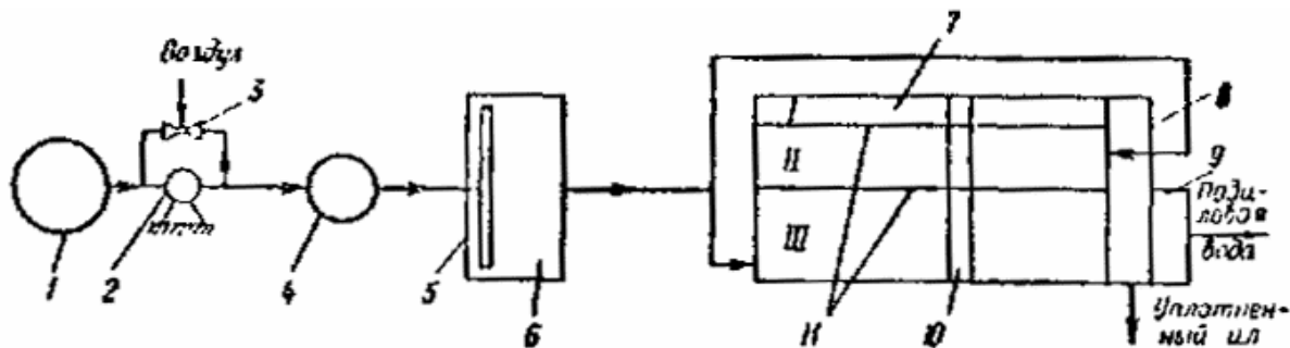
Рис. 22. Схема флотационного уплотнителя избыточного активного ила (ИАИ)
