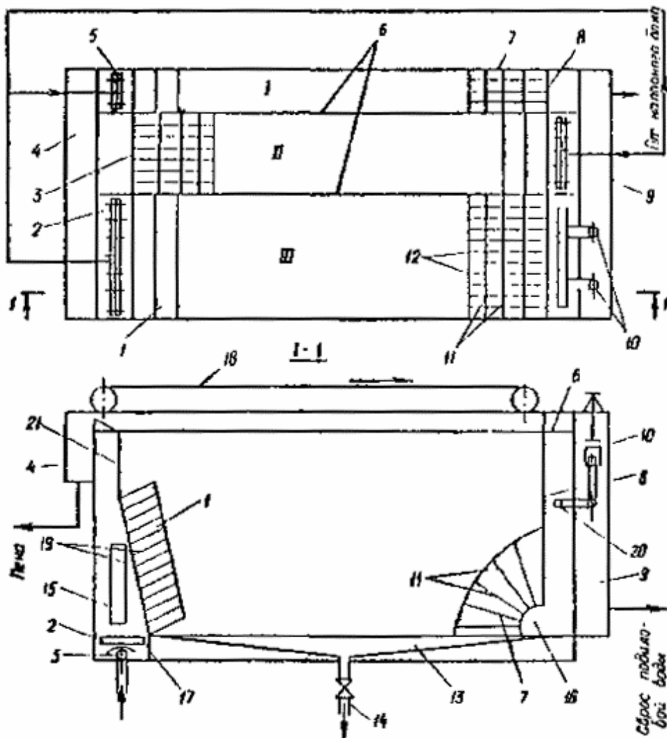
Рис. 21. Схема флотационного илоуплотнителя
