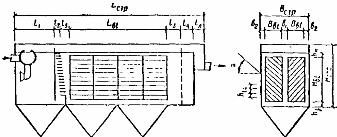
Рис. 3. Схема тонкослойного отстойника, работающего по перекрестной схеме удаления осадка где h_3 - высота, необходимая для расположения рамы, на которой устанавливаются блоки ( h_3 = 0,2-0,3 м; h_m = 0,1 м).
