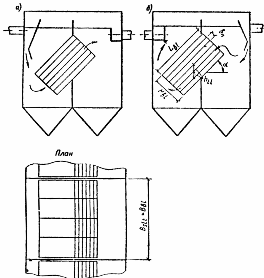
Рис. 4. Схема тонкослойного отстойника, работающего по противоточной схеме удаления примесей а - тяжелых примесей; б - легких примесей (масла, нефтепродукты и т. а.)
