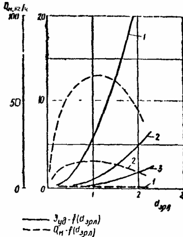
Рис. 15. Зависимость удельных энергзатрат и производительности по кислороду от диаметра эрлифтных аэраторов при различных значениях интенсивности аэрации 1 - J_a = 5 ; 2 - J_a = 10 ; 3 - J_a = 15 \text{ м}^3/(\text{м}^2\cdot\text{ч})
