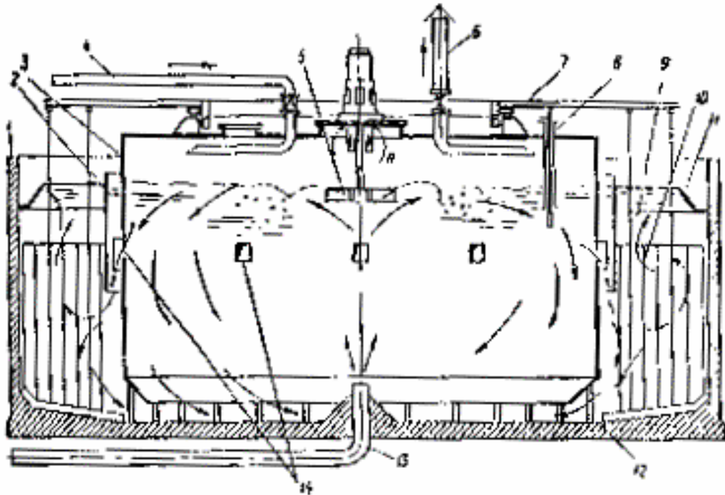
Рис. 16. Схема окситенка
