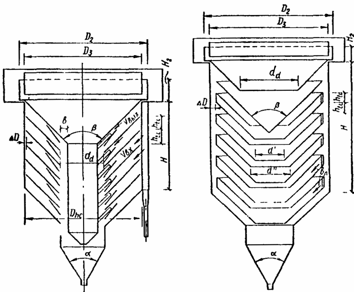
Рис. 8. Схема многоярусного гидроциклона с центральными отбором очищенной воды
