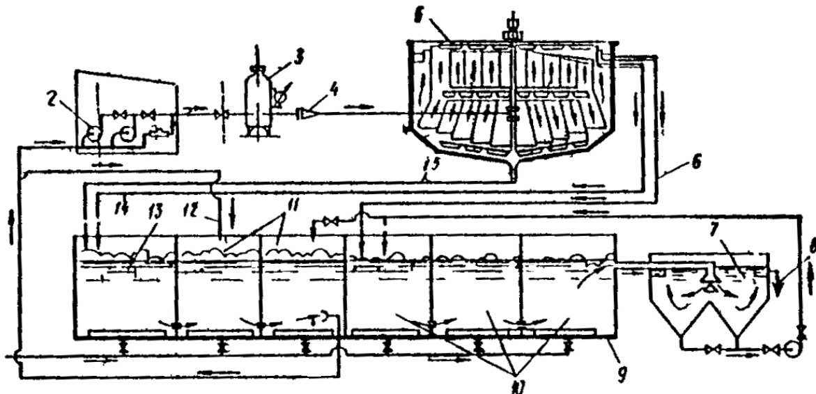
Рис. 17. Схема аэротенка с флотационным илоотделителем для очистки производственных сточных вод
