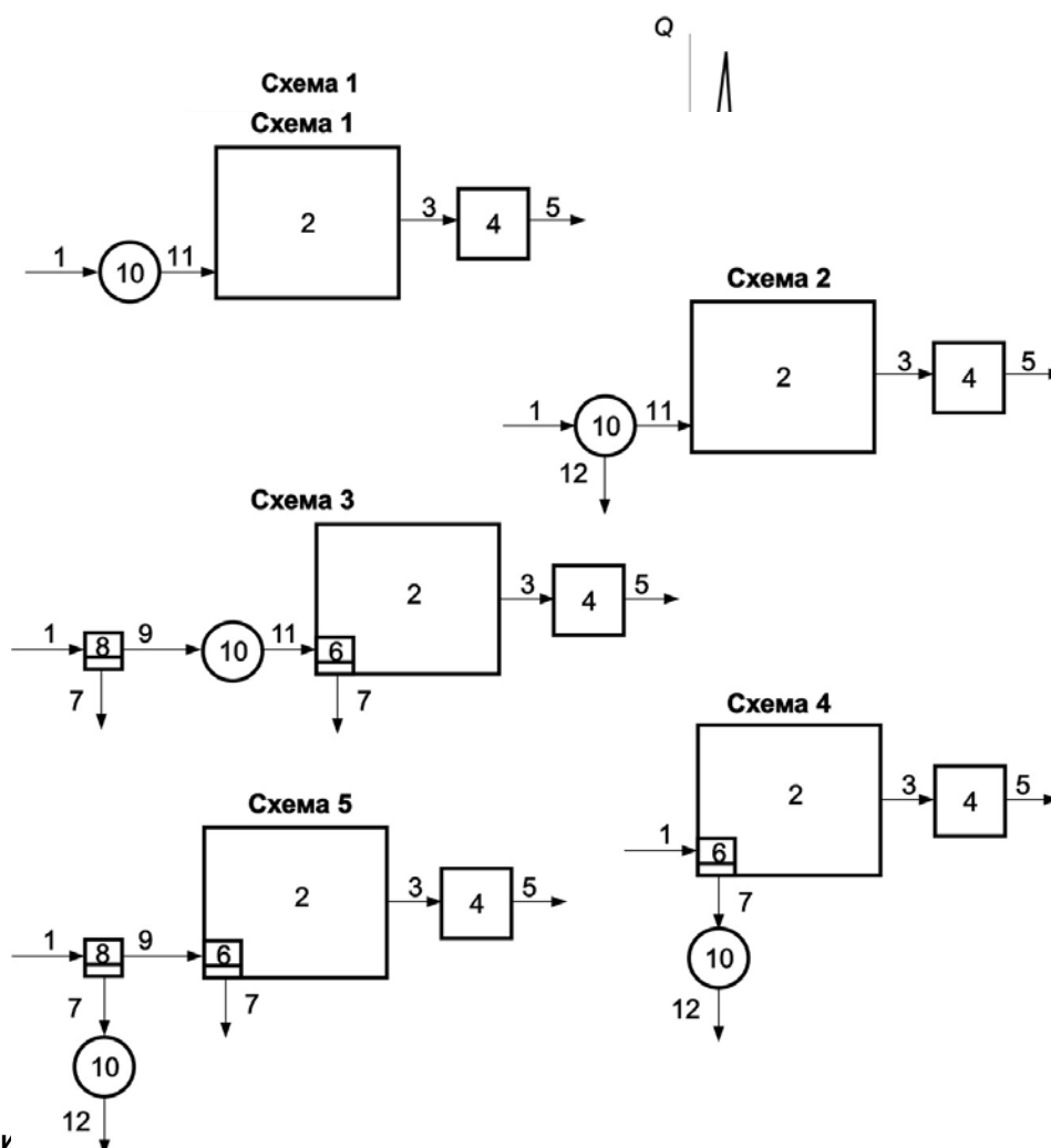
Рис. 2. Основные схемы перекачки дождевого стока
