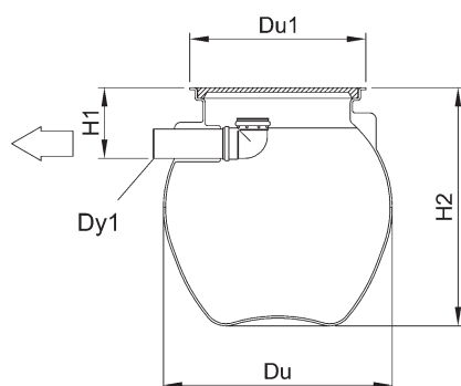
рис. 4.5 в (HEK 200 LK)
