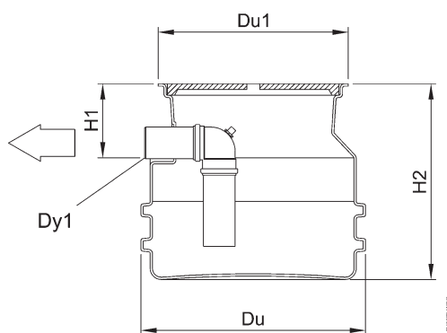
рис. 4.6 а (MiniPEK A 0,2)
