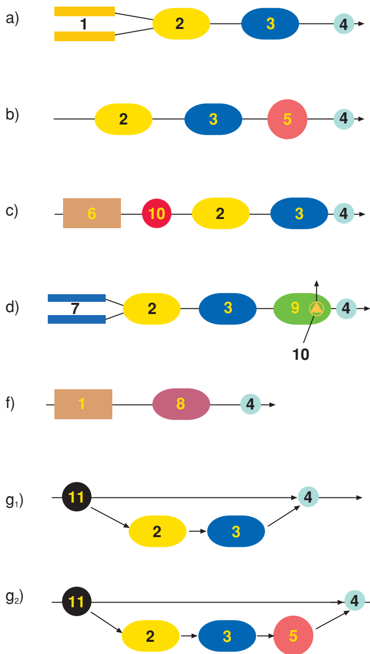
Рис. 3.1 Принципиальные технологические схемы с использованием локальных очистных сооружений "Wavin-Labko".
