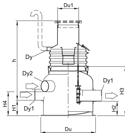
рис.4.21 б (EuroNOK FRW)
