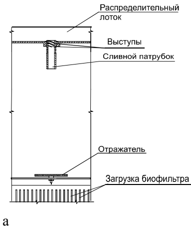
а б Рис. 7.7. Система орошения
