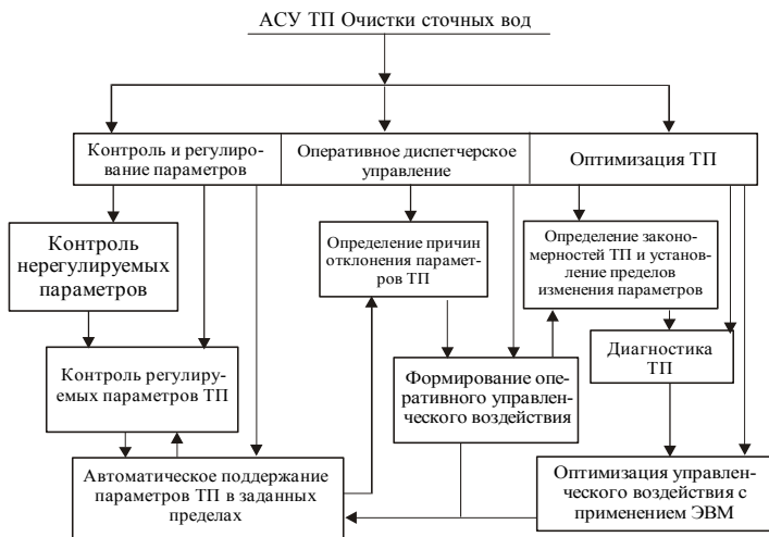
Рис.11.16 - Структурная схема автоматической системы управления технологическим процессом очистки сточных вод.
