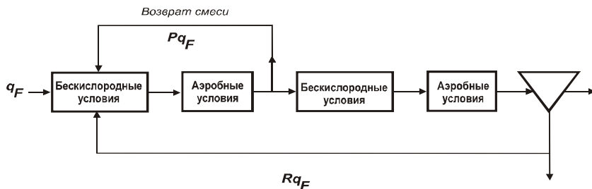
Рис 6.3. Схема Барденпо для удаления соединений азота.
