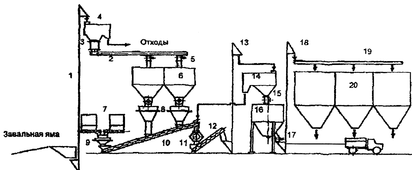
Рисунок Г.5. Технологическая схема приготовления кормосмесей с использованием местного сырья
