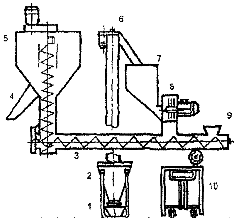
Рисунок Г.6. Схема технологического процесса приготовления комбикормов
