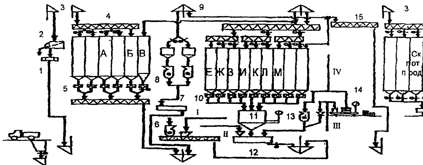
Рисунок Г.1. Принципиальная схема технологического процесса производства комбикормов и БВД
