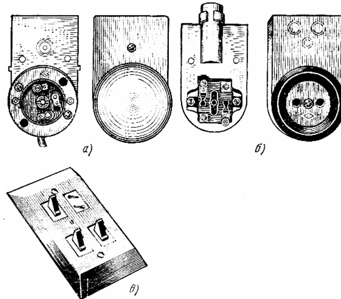
Рис.2. Подпотолочный выключатель (а), надплинтусная штепсельная розетка (б), блок с выключателями и штепсельной розеткой (в)
