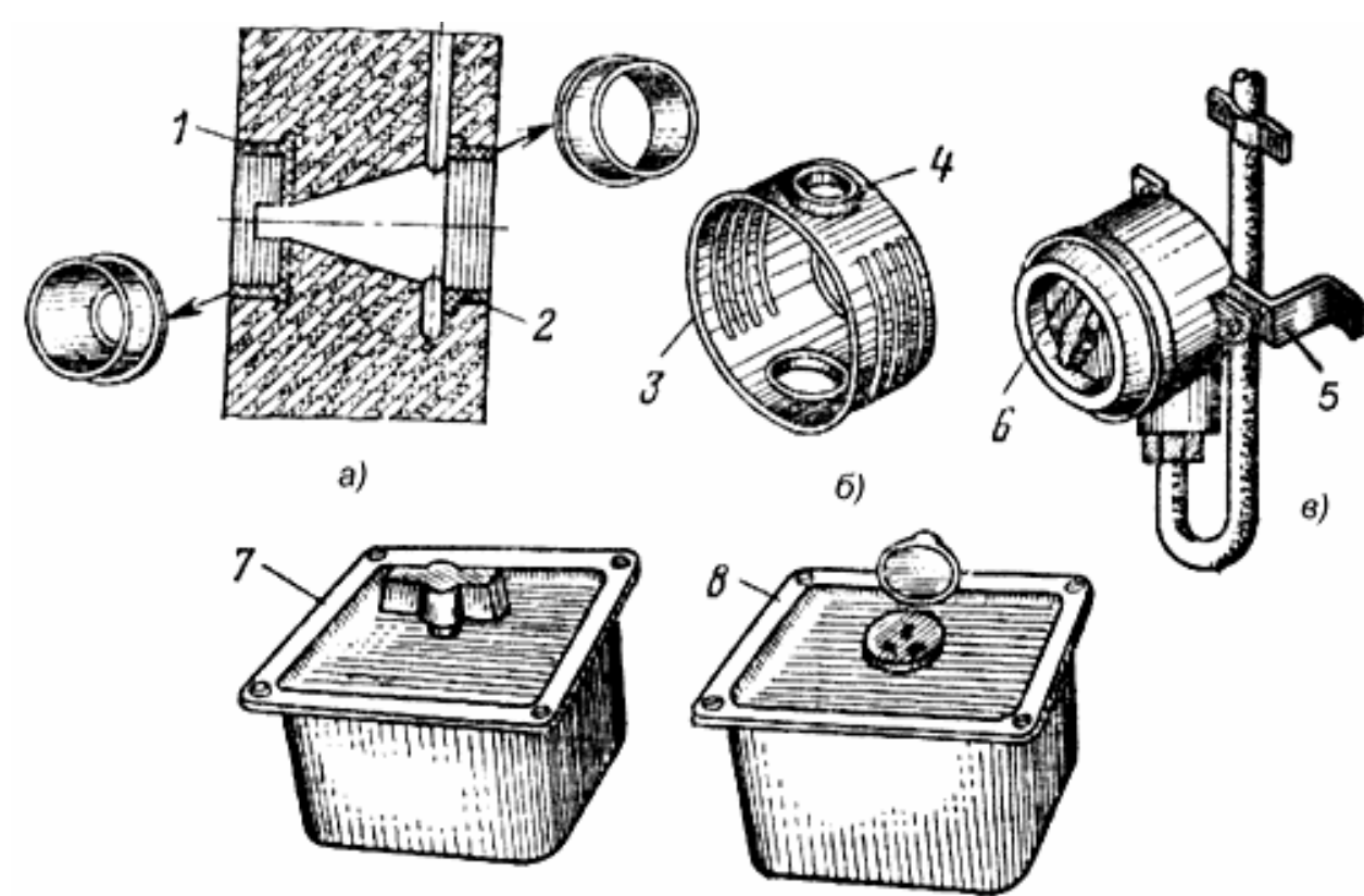
Рис. 1.Крепление электроустановочных изделий: а -распорными лапками в замоноличенных коробках Л90 и Л91; б - распорными лапками в коробках КУВ-1М; в - открыто на скобах К130; г -в коробках КВ и КР; 1 - коробка Л91; 2 - коробка Л90; 3 -коробка КУВ-1М; 4 -втулка пластмассовая; 5 -скоба К130; 6 - выключатель полугерметический; 7 - коробка КВ со встроенным выключателем; 8 - коробка КР со встроенной розеткой
