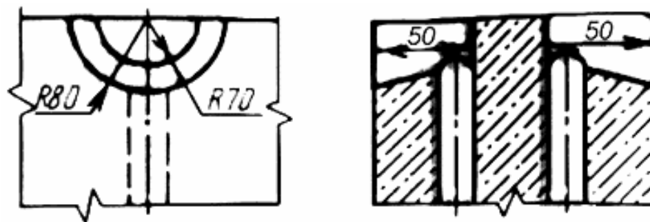
Рис.7. Протяжные ниши в стеновых железобетонных межквартирных панелях
