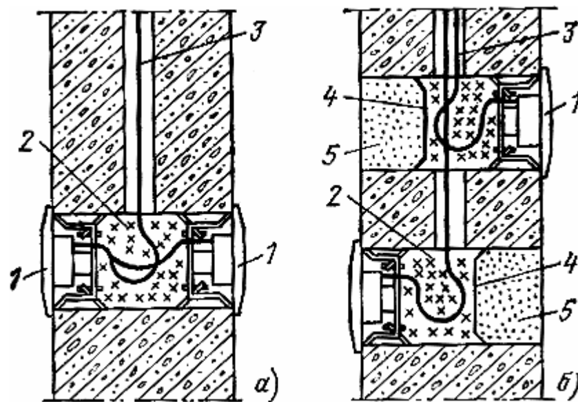
Рис.14. Узлы установки штепсельных розеток в стеновых панелях для межкомнатной перегородки (а) и для межквартирной перегородки (б): 1 - штепсельная розетка; 2 - негорючий минераловатный наполнитель; 3 -провода; 4 -круглая стальная заглушка; 5 -заделка цементным раствором
