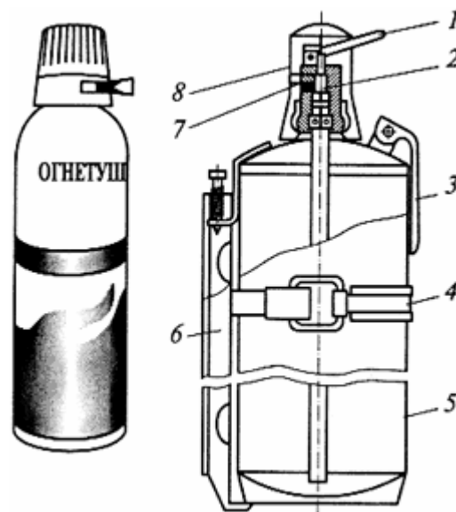
Рис.29. Хладоновый огнетушитель ОУБ-ЗА (ОУБ-7А):
