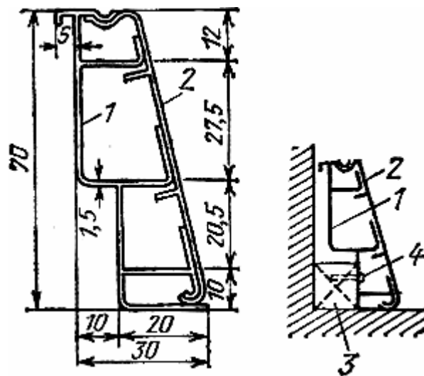
Рис.20. Электроплинтус: 1 - корпус; 2- крышка; 3- раскладка; 4 -шуруп
