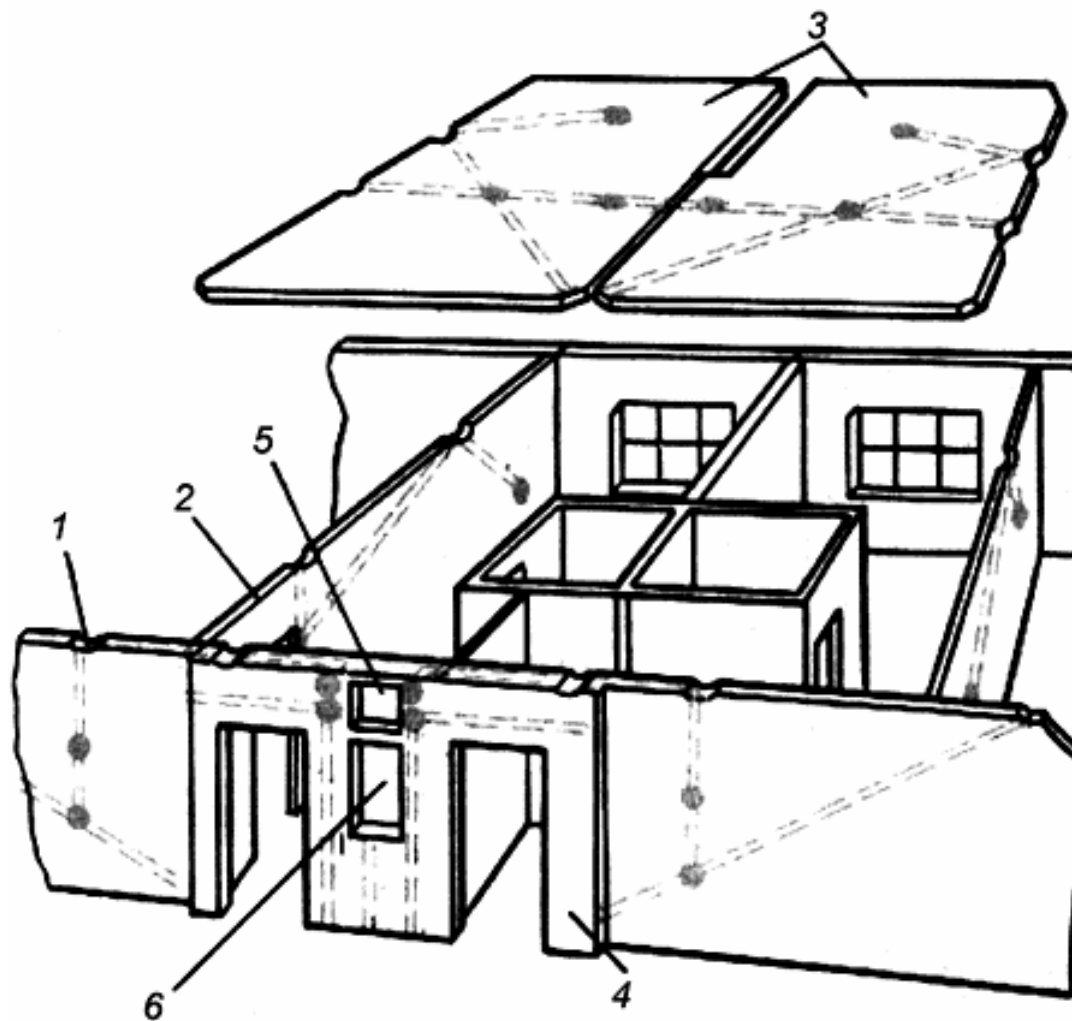
Рис.5. Скрытые электропроводки в каналах:
