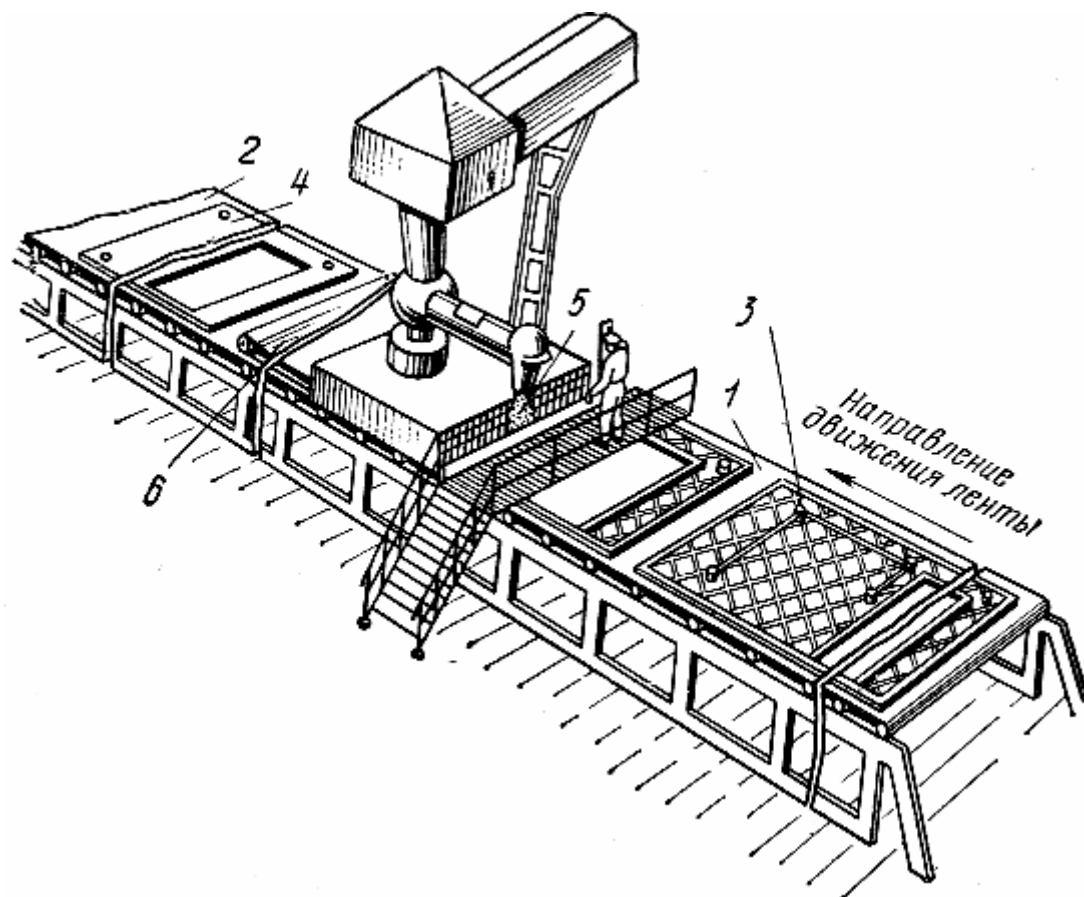
Рис.18. Изготовление гипсобетонной перегородки с замоноличенной электропроводкой на прокатном стане: 1- приемный рольганг; 2- выходной рольганг; 3- деревянный каркас панели с закрепленной на нем проводкой; 4- отформованная панель; 5 - зона заполнения каркаса гипсобетонным раствором; 6- зона проката (формования)
