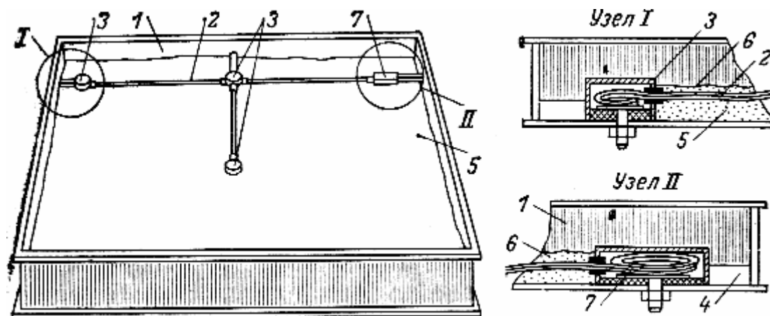
Рис.19. Замоноличивание заготовки электропроводки в стеновую шлакобетонную панель:
