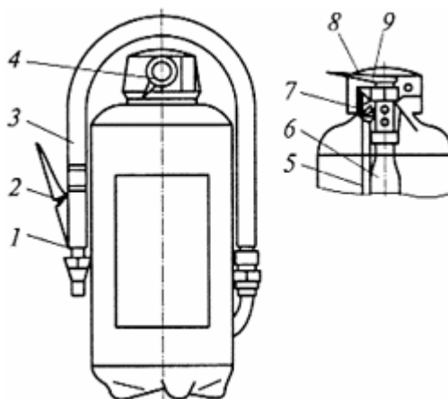
Рис.52. Ручной порошковый огнетушитель ОП-5:
