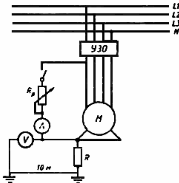
Рис.44. Схема проверки УЗО по методу 3.
