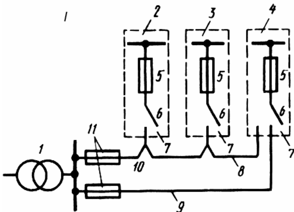
Рис.1. магистральная петлевая схема (I)
