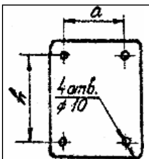
Рис.39. Размеры для открытого крепления щитков
