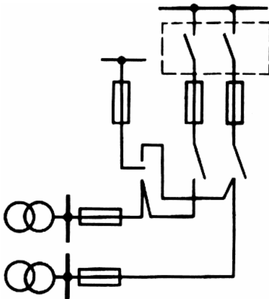
Рис.6. Схемы питания жилых 17-25-этажных домов и более
