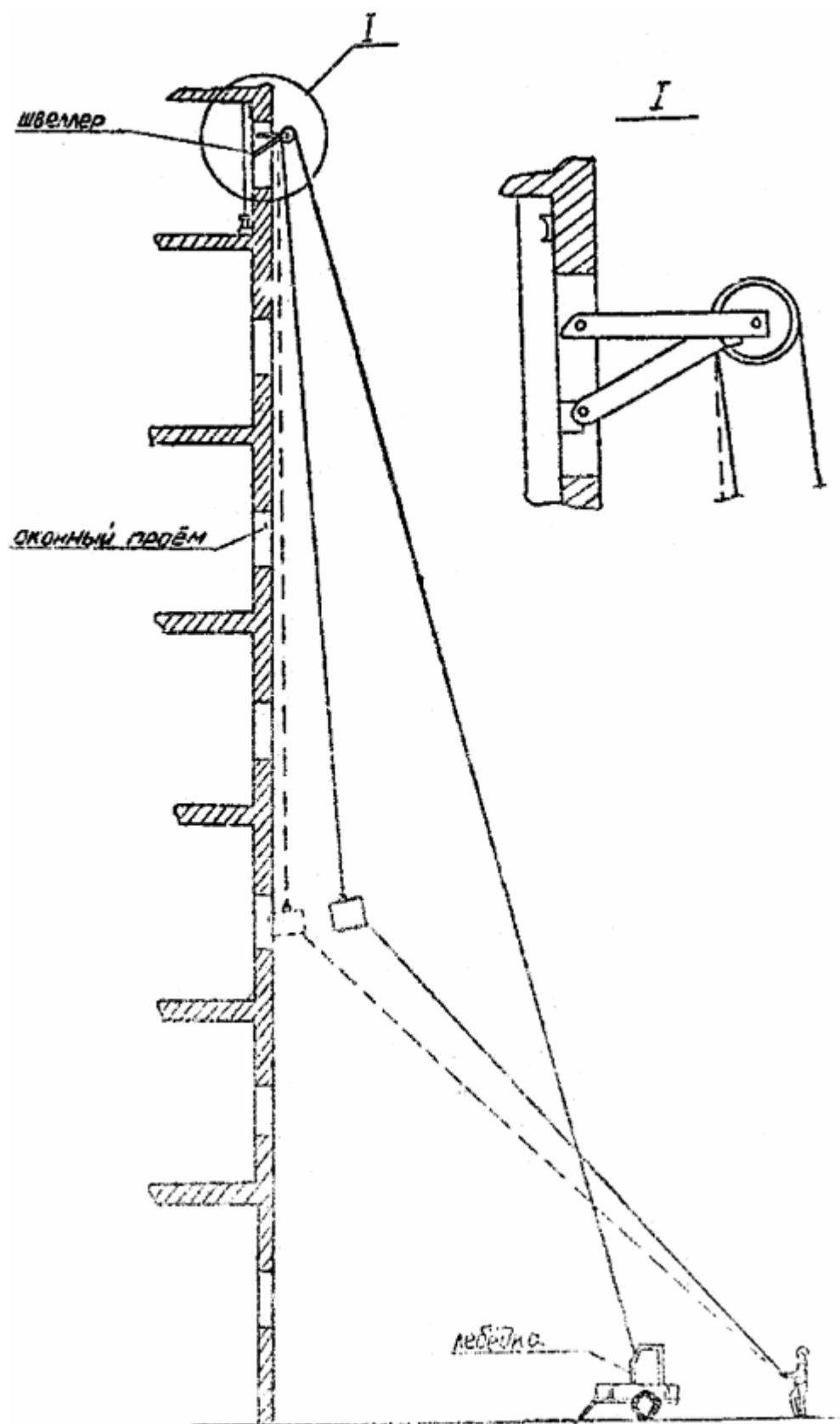
Рис.38. Схемы подъема груза в контейнерах
