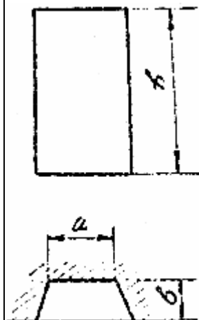
Рис.36. Размеры ниш для установки осветительных групповых и квартирных щитков
