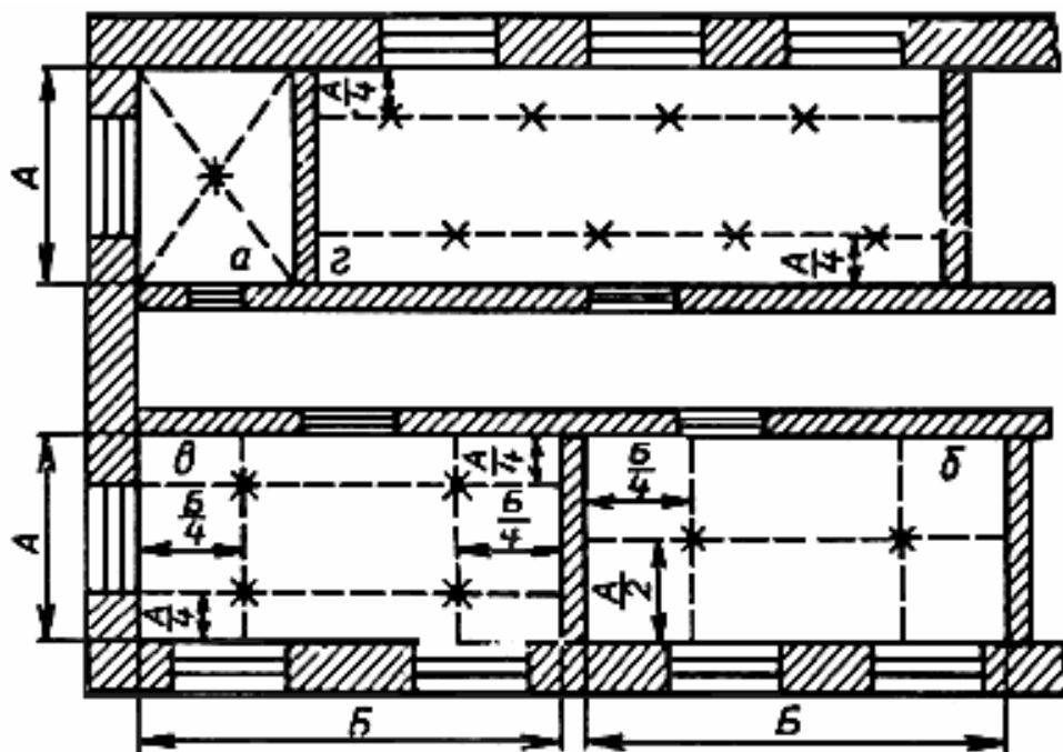
Рис.40. Разметка мест установки светильников в помещениях
