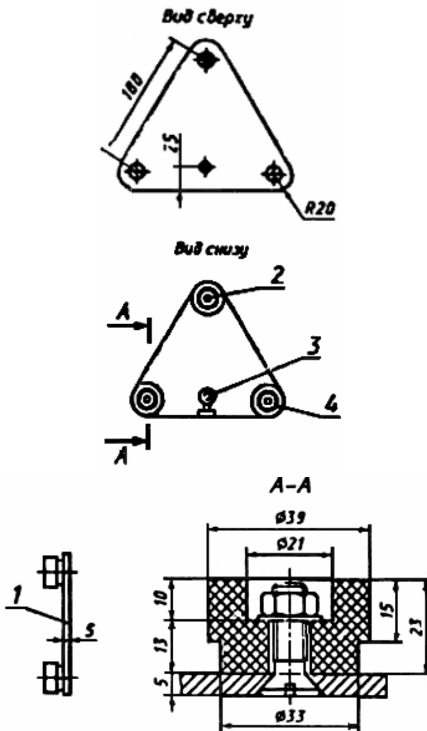
Рис.45. Испытательный электрод 2
