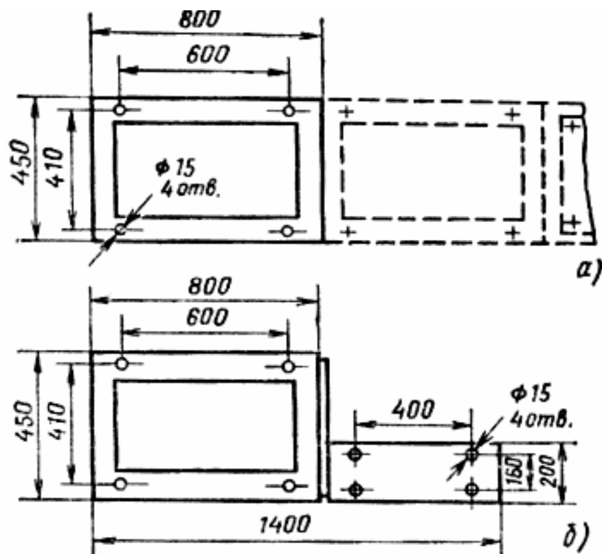
Рис.32. Установочные размеры вводных панелей
