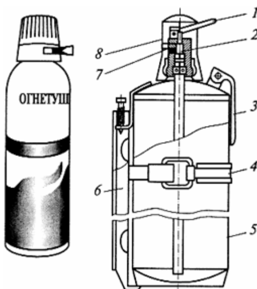
Рис.51. Хладоновый огнетушитель ОУБ-3А (ОУБ-7А):
